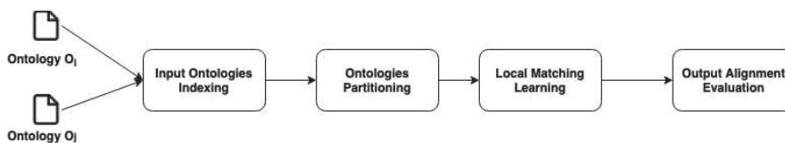
Fig. 1. POMap++ overview
