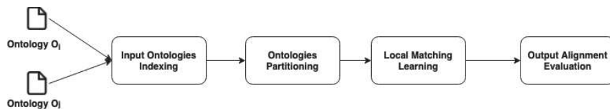
Fig. 1. POMap++ overview
