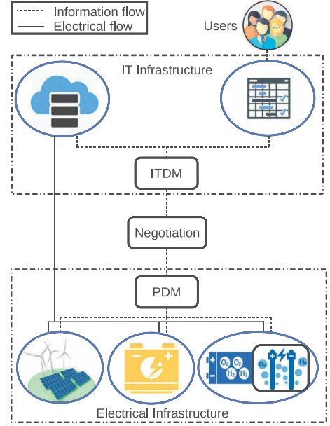
Fig. 1. Datacenter model.
