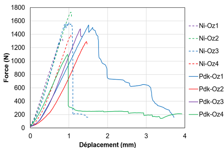
Fig. 3 : Courbe Force déplacement (essai de traction)
