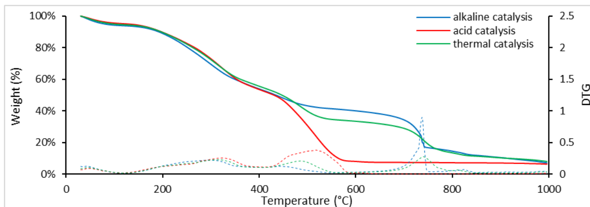
Fig. 1. Analyse thermogravimétrique.
