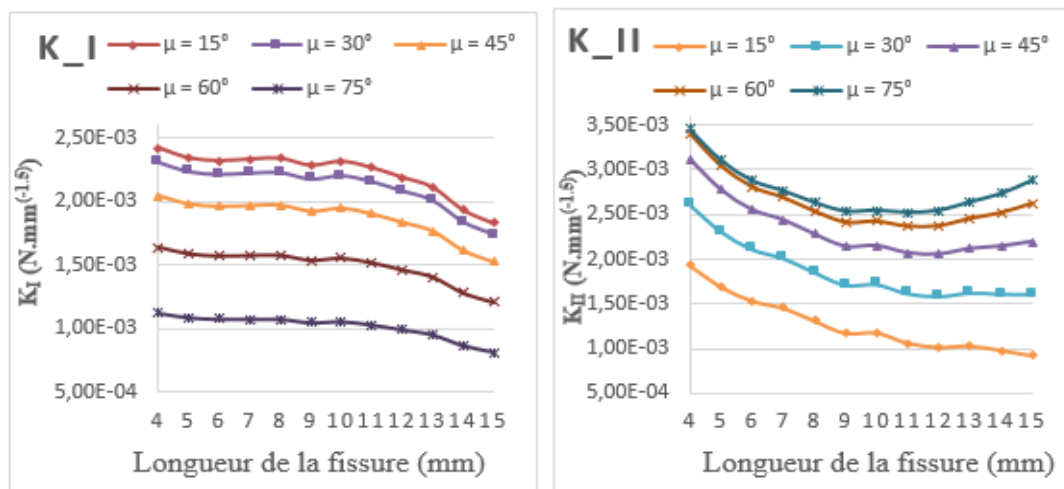
Fig. 3 : Facteur d'intensité de contraintes en fonction de la longueur de fissure.
