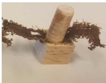
Fig.2 : Echantillon soudé : P_s=6\text{MPa} , v=0.44\text{m.s}^{-1} .
