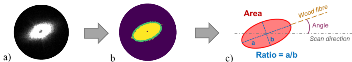
Fig. 1 : a) Image en niveaux de gris de la diffusion d'un laser sur une surface de bois. b) Binarisation et fit ellipse . c) Schéma d'une ellipse avec l'aire, le ratio et l'angle.
