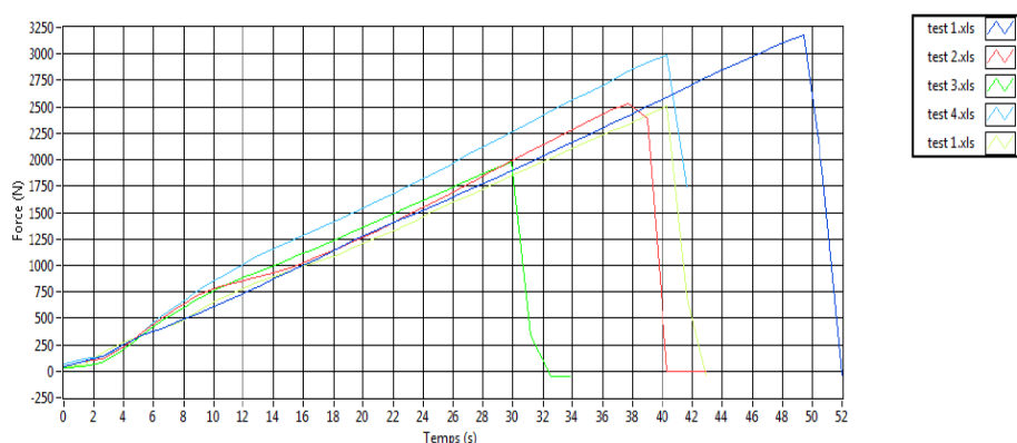
Fig.3 : Evaluation de la qualité de collage des panneaux de contreplaqués collés avec des colles écologiques.
