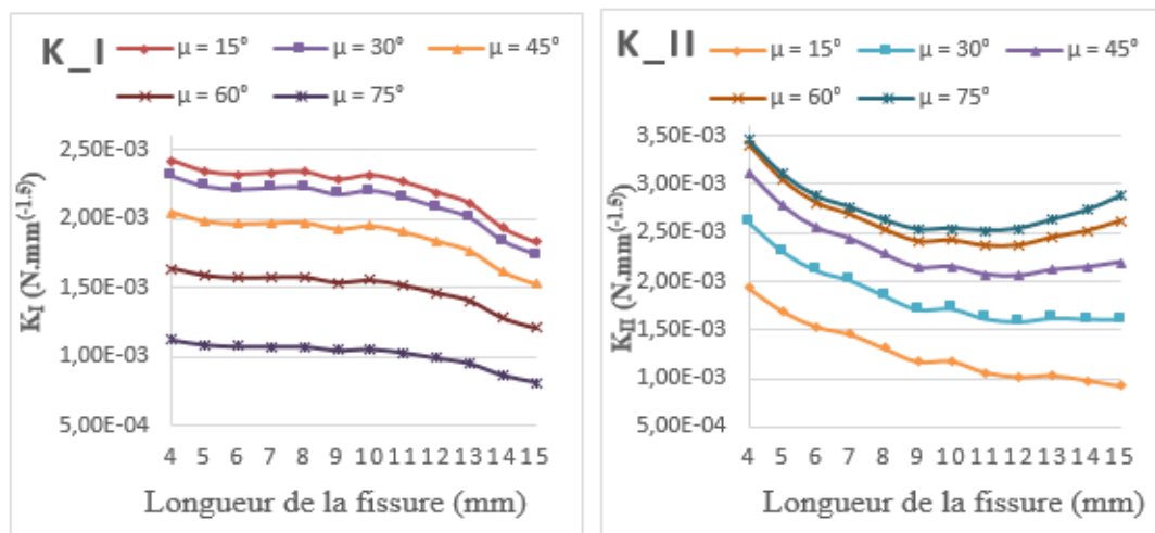
Fig. 3 : Facteur d'intensité de contraintes en fonction de la longueur de fissure.
