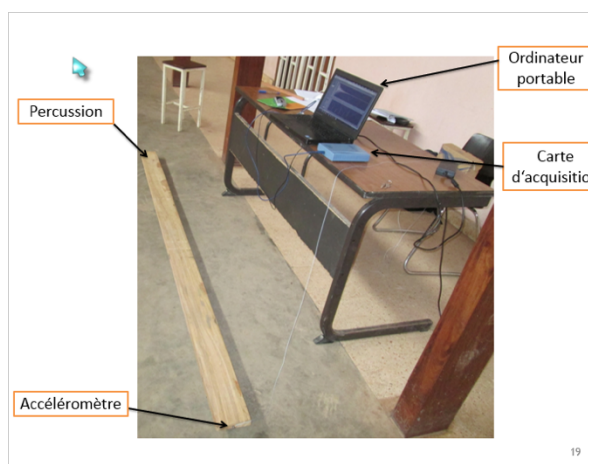
Fig. 1 : Essai vibratoire
