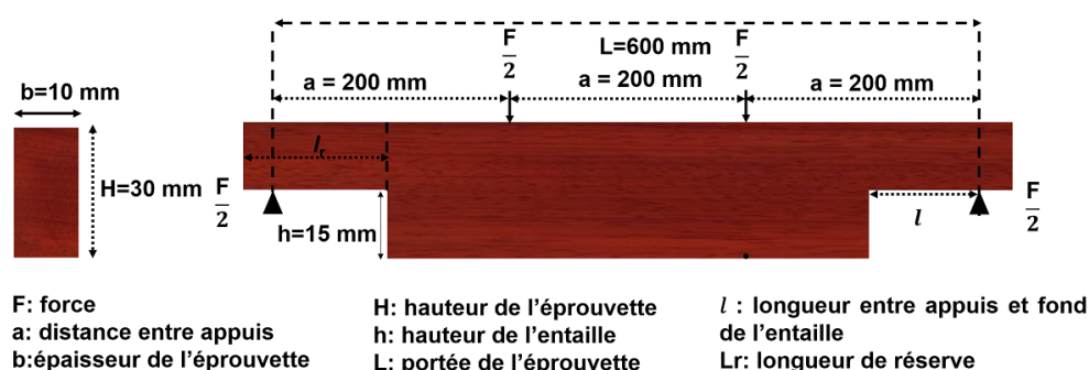
Fig. 1 : Configuration des éprouvettes entaillées pour les essais de fluage en extérieur abrité
