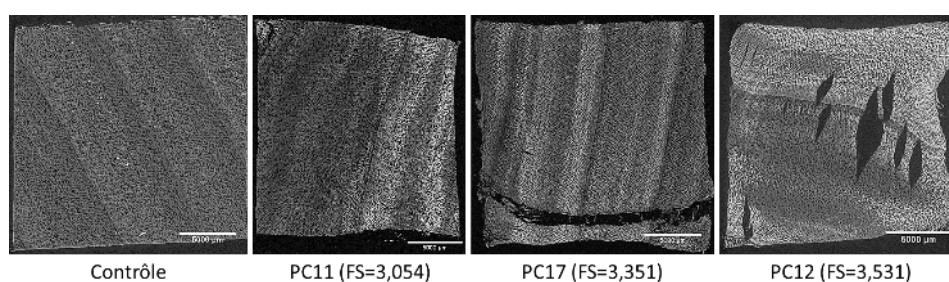
Fig1. Tomographies rayons X des échantillons prétraités par explosion de vapeur. Les coupes transversales sont représentées.
