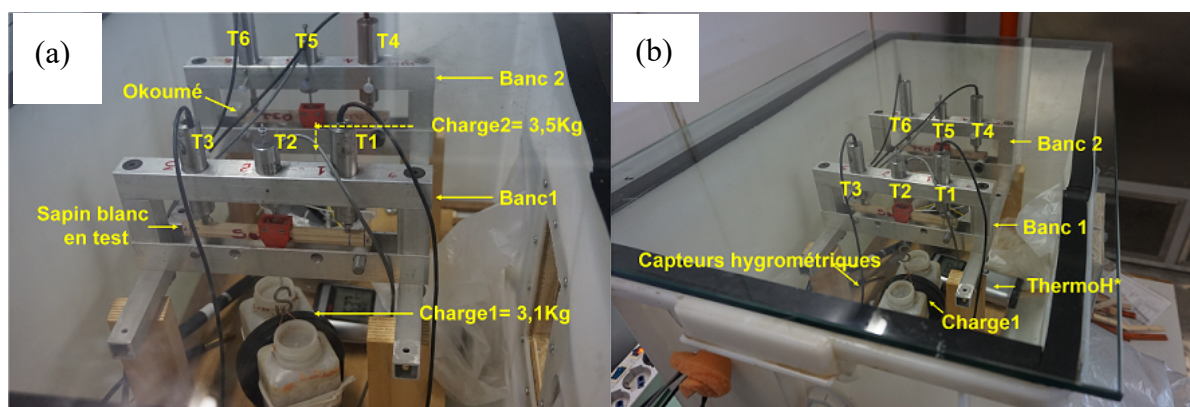
Fig. 4: Banc de fluage : (a) mise en charge de deux éprouvettes, Sapin et Okoumé ; (b) boîte de conditionnement
