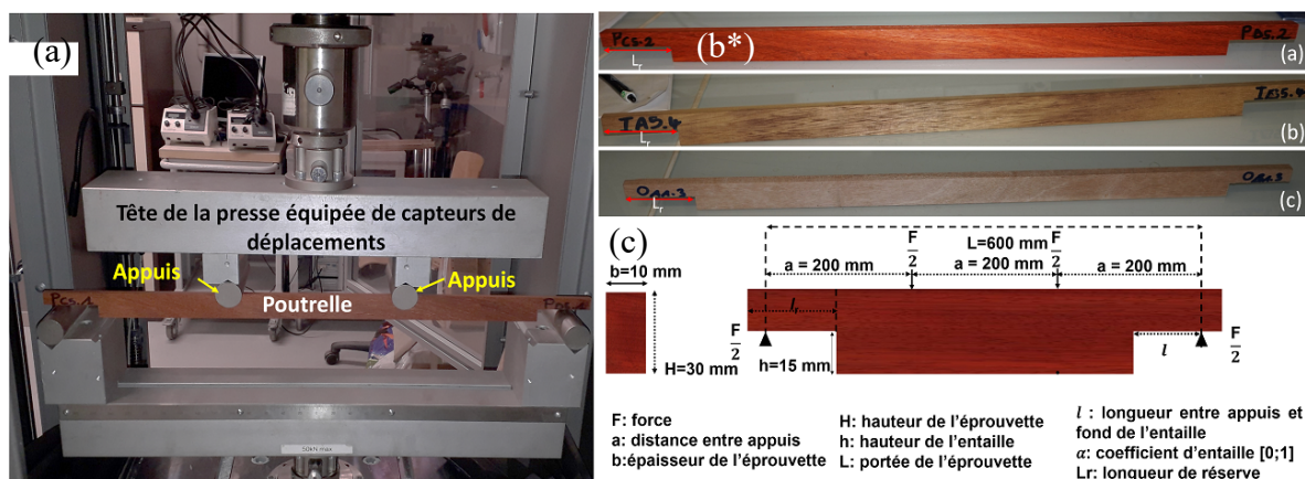
Fig. 1 : Essais de rupture : (a) dispositif expérimental avec presse Zwick/Roell ; (b) poutrelles entaillées testées (a : Padouk ; b : Iroko ; c : Okoumé) ; (c) géométrie des poutrelles entaillées.
