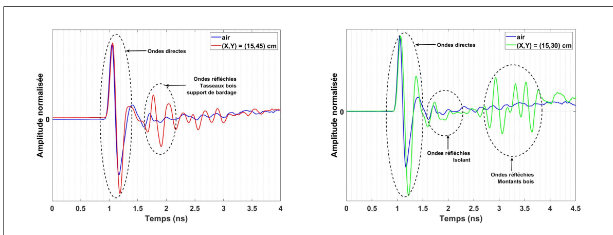
Fig. 3 : Mesure par une antenne dans l'air (à gauche) et sur la paroi de la maquette du mur à ossature bois (à droite)
