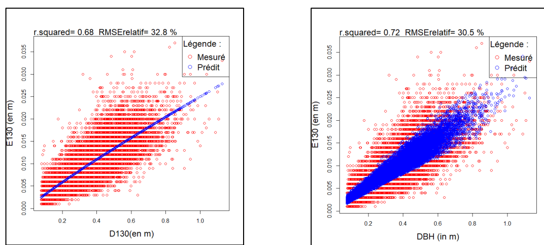
Fig. 2 : Résultats des modèles : E130 = a \cdot D130^b (à gauche) et E130 = (a \cdot alt + b) \cdot D130^c (à droite)
