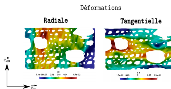
Fig. 2 : Champs de déformations radiale et tangentielle pour une éprouvette mise en présence d'un solvant mixte Eau-DMF (75%-25%)
