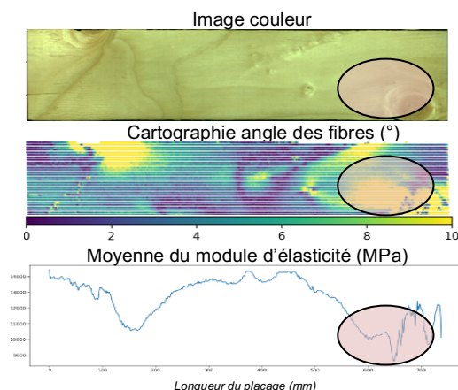
Fig. 2 : Estimation du module d'élasticité suivant la longueur du placage
