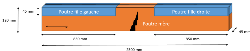
Figure 1 : Schéma de découpe des poutres filles dans les poutres mères testées
