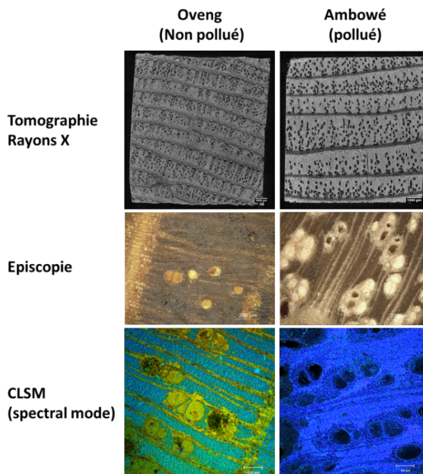
Fig.4. Observations réalisées en tomographie rayons X, microscopie à épiscopie et microscopie confocale sur les échantillons de bois d'Oveng (site non pollué) et d'Ambowé (site pollué).
