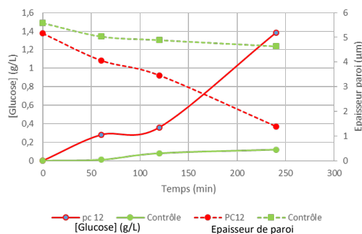
Fig 5. Evolution de la production de glucose et de l'épaisseur pariétale dans des échantillons de peuplier contrôle et explosés à la vapeur.
