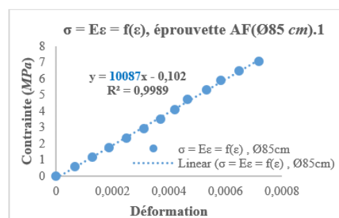
Fig. 2 : Régression linéaire contrainte/déformation de détermination du module d'élasticité en flexion 4-points de l'éprouvette AF(Ø85).1 pour le diamètre 85cm
