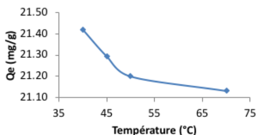
Fig. 3 : Effet de la température sur l'élimination du bleu de méthylène (100ppm) par les coques de Lophira lanceolata
