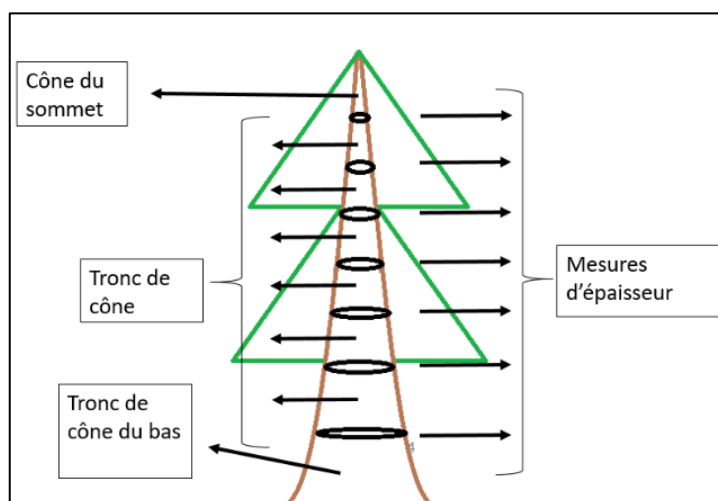
Fig. 1 : Schéma de modélisation d'une tige modélisée par une suite de tronc de cône
