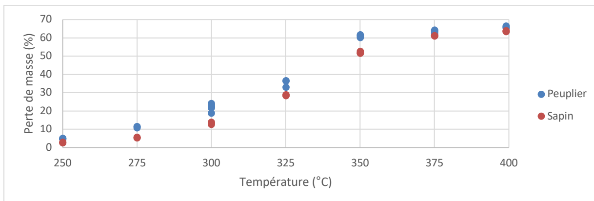
Fig. 3 : Perte de masse du peuplier et du sapin en fonction de la température de traitement. Pour chaque température, trois échantillons d'une même essence sont testés simultanément.
