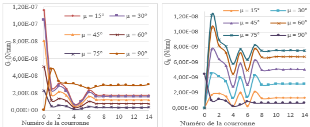
Fig. 2 : Indépendance du contour d'intégration de G_I et G_{II} en fonction de l'angle \mu .
