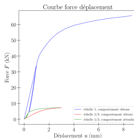
Fig. 5 : Courbe expérimentales force déplacement des assemblages
