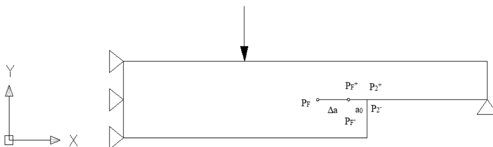
Fig. 2 : Propagation de la fissure dans le cas d'étude.
