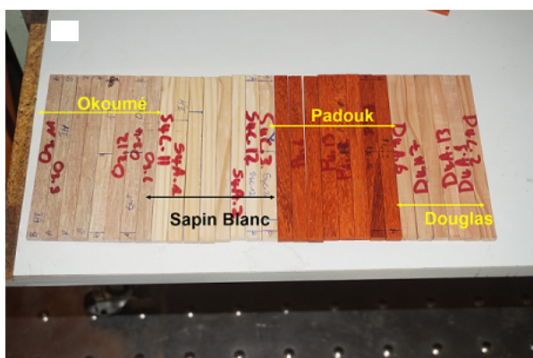
Fig. 2 : Epreuves non entaillées pour les essais de fluage en ambiance contrôlée
