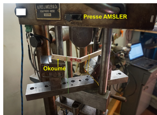
Fig. 3 : Essais de rupture sur éprouvettes appariées
