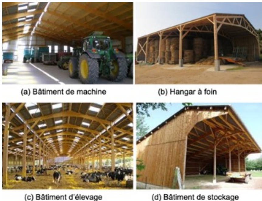
Fig. 1 : Exemples de bâtiments agricoles
