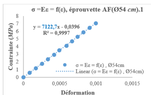
Fig. 1 : Régression linéaire contrainte/déformation de détermination du module d'élasticité en flexion 4-points de l'éprouvette AF(Ø54).1 pour le diamètre 54 cm
