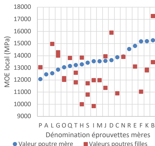
Figure 7 : Valeurs de modules élastiques locaux en flexion des corps d'éprouvettes parents et enfants
