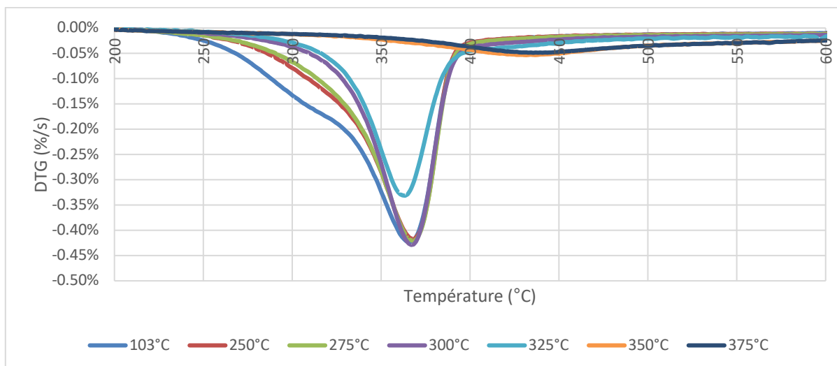
Fig. 5 : DTG du peuplier. Valeurs pour un échantillon non traité (103°C) et pour différentes températures de traitement.
