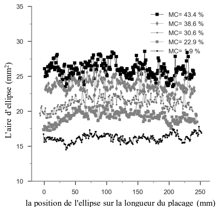
Fig 1. Exemple de distribution de l'aire de l'ellipse à différents taux d'humidité sur toute la longueur d'un placage de hêtre de 1 mm d'épaisseur
