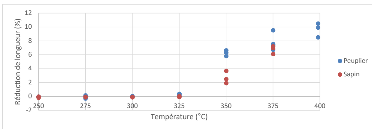
Fig. 4 : Réduction de longueur du peuplier et du sapin en fonction de la température de traitement. Pour chaque température, trois échantillons d'une même essence sont testés simultanément.
