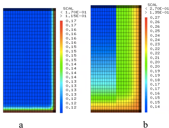
Fig. 3 : Exemple de champs hydriques dans la poutre bois pour a) fin de l'année 1, b) fin de l'année 10
