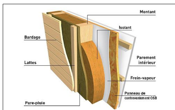
Fig. 1 : Schéma de la maquette du mur à ossature bois (FCBA-Bordeaux)
