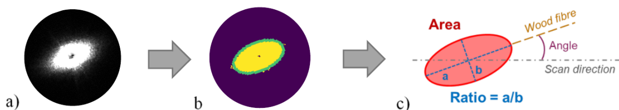
Fig. 1 : a) Image en niveaux de gris de la diffusion d'un laser sur une surface de bois. b) Binarisation et fit ellipse . c) Schéma d'une ellipse avec l'aire, le ratio et l'angle.
