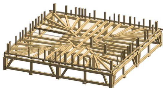
Fig. 4 : Vue 3D de l'enrayure supportant l'étage
