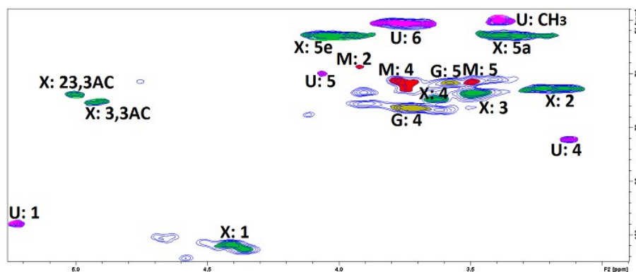
Fig. 4: RMN 2D HSQC des hémicelluloses extradites par explosion à la vapeur : X: xylose; M: mannose; G: glucose; U: 4-O-méthyle- \alpha -D-glucuronique; AC: acétyle.
