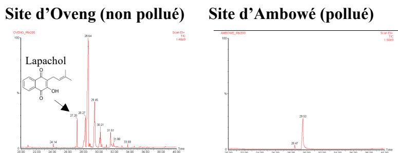
Fig. 5. Chromatogramme GC-MS des bois d' A. germinans issus du site non pollué d'Oveng et pollué d'Ambowè.
