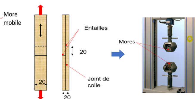
Fig. 2 : Eprouvette et dispositif de l'essai de cisaillement
