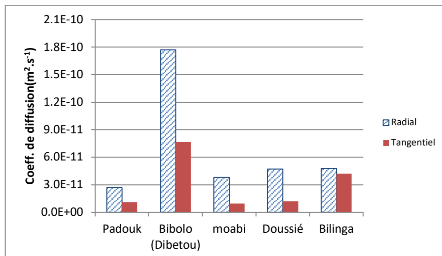
Fig. 2 : Coefficient de diffusion d'eau liée
