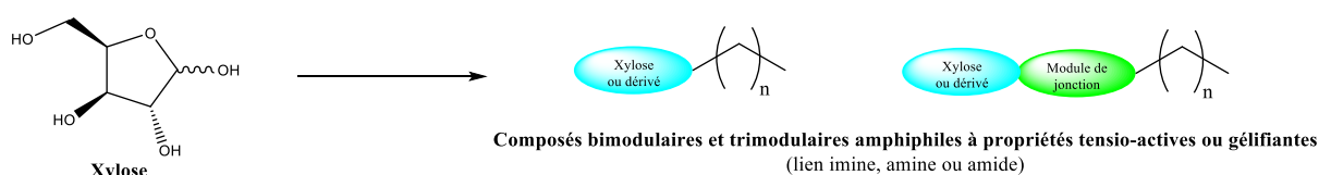
Fig. 1 : Composés cibles
