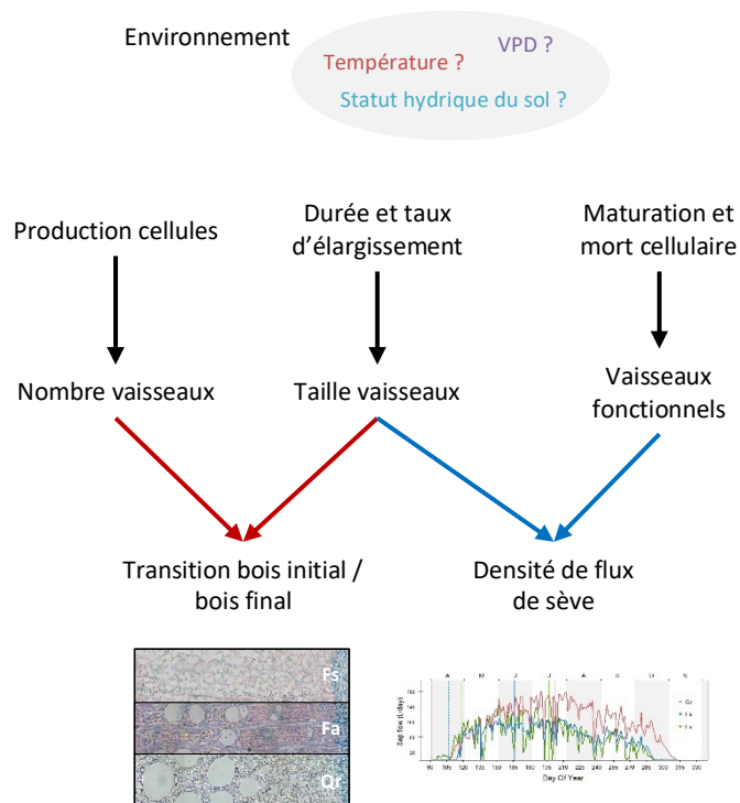
Fig. 1 : Résumé graphique
