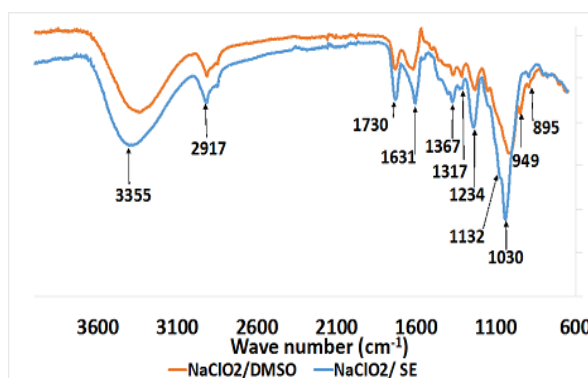
Fig.2 : Analyse IRTF
