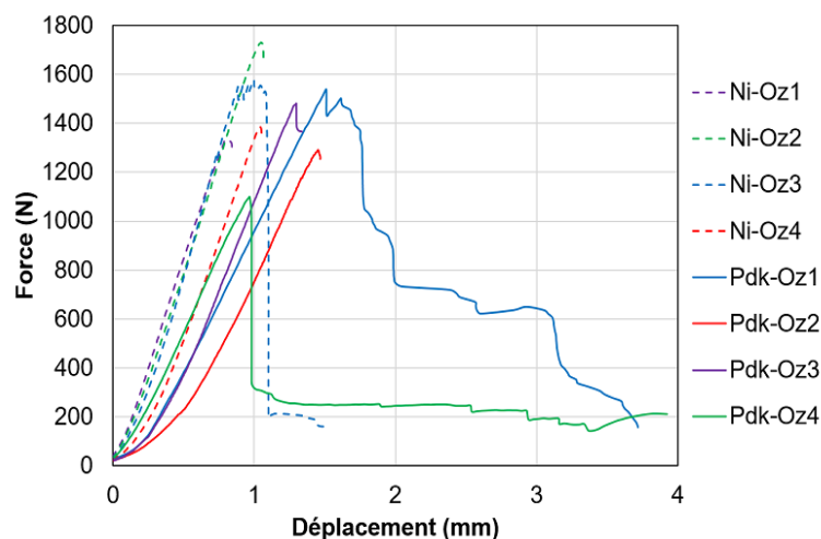
Fig. 3 : Courbe Force déplacement (essai de traction)
