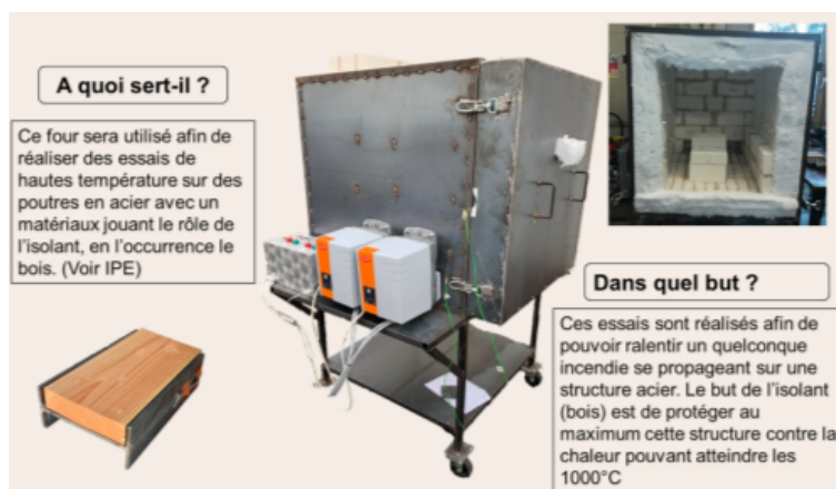
Fig. 1 : Four d'essai
