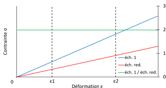
Fig. 2 : Lois de comportement linéaires
