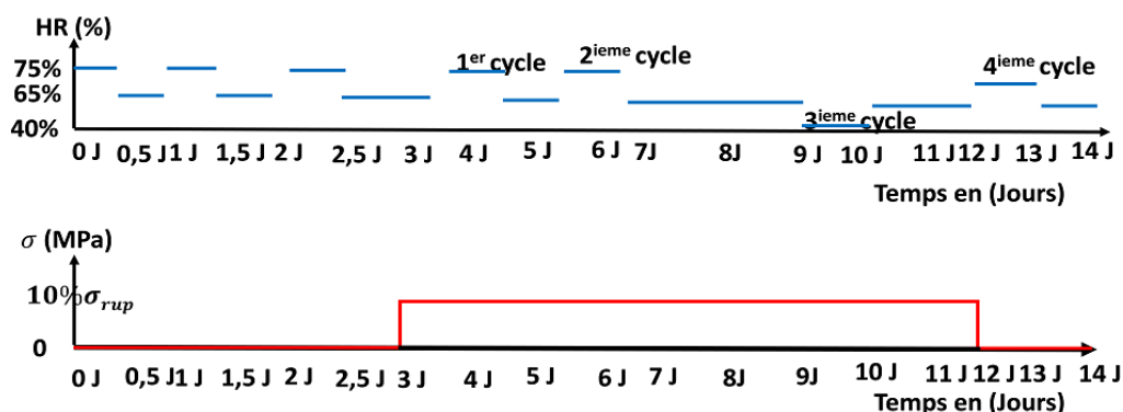
Fig. 5 : Planning de chargement hydro-mécanique
