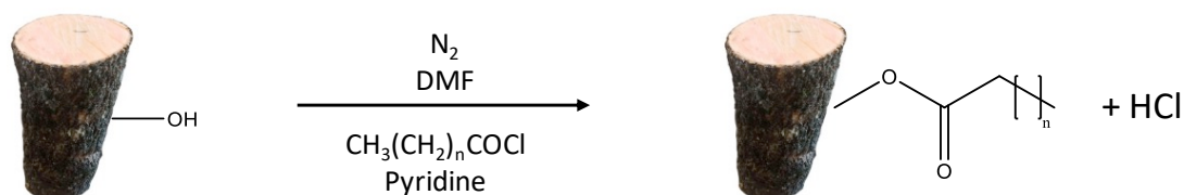
Fig. 2 : Acylation du bois avec un chlorure d'acide gras
