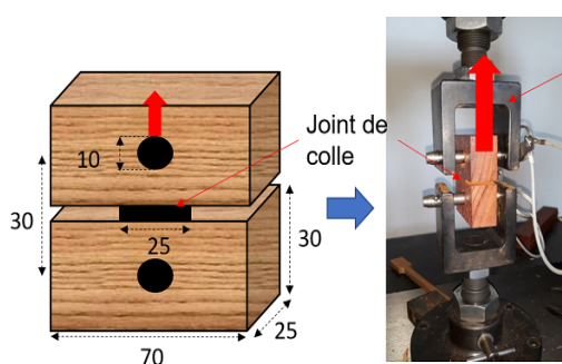
Fig. 1 : Eprouvette et dispositif de l'essai de traction pure
