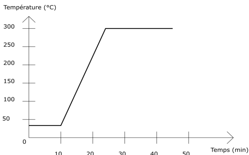
Fig. 1 : Programme de montée en température du réacteur. Exemple pour l'expérience à 300°C.
