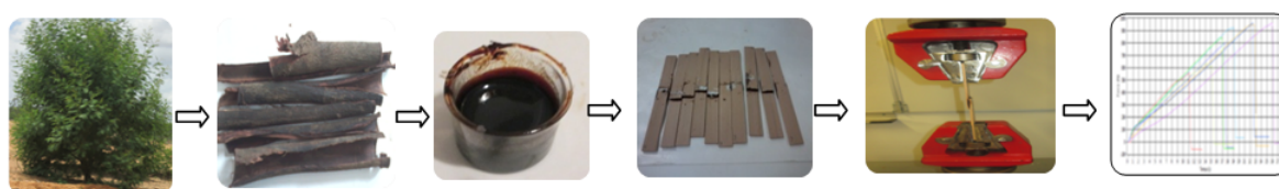
Fig.2 : Protocole de préparation des panneaux de contreplaqués collés avec des colles écologiques de tanin d' Acacia mollissima .
