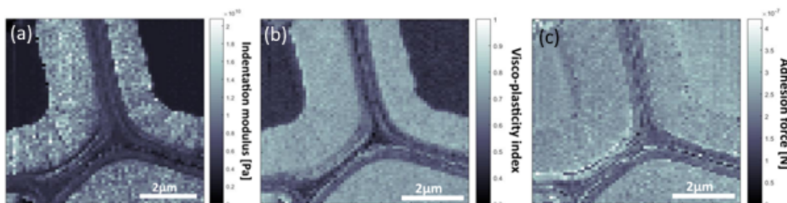
Figure 3 : Cartographies des modules d'indentation, de l'indice de viscoplasticité et de la force d'adhésion à l'intersection de trois fibres de peuplier (résolution 100nm).
