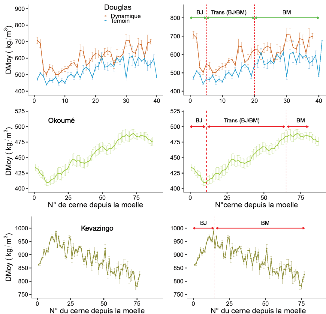
Fig. 4 : Profils des variations radiales de la densité moyenne des cernes du Douglas de l'Okoumé et du Kevazingo. Les barres d'erreur représentent la variabilité induite par l'effet arbre (n= 5 arbres). Les lignes rouges marquent les limites qui correspondent visuellement aux phases de transition. DMoy = densité moyenne des cernes.
