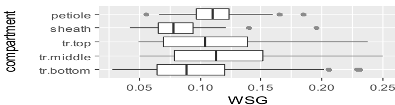
Fig. 3 : Variation de l'infradensité selon le compartiment
