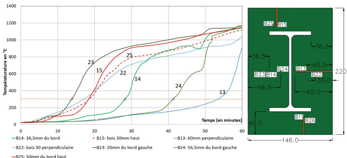
Fig. 6 : Mesures et position des thermocouples dans le bois
