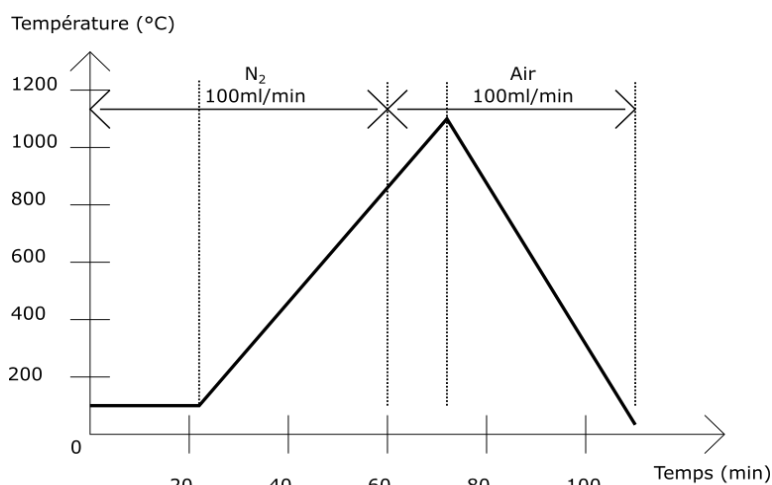
Fig. 2 : Programme de traitement pour l'analyse thermogravimétrique.
