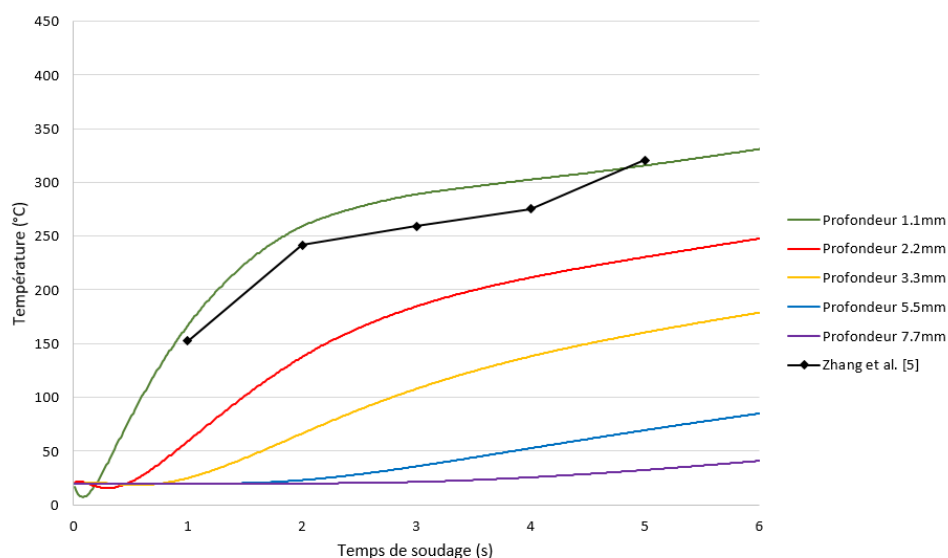
Fig.3 : Comparaison des courbes d'évolution de la température à différentes profondeurs obtenues par le modèle numérique et un résultat obtenu dans la littérature (Zhang 2017)
