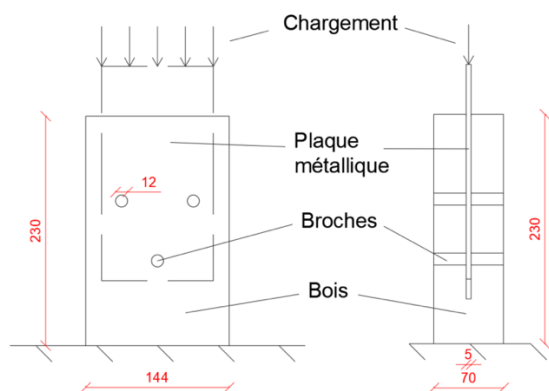
Fig. 4 : Assemblages testés (échelle 1)
