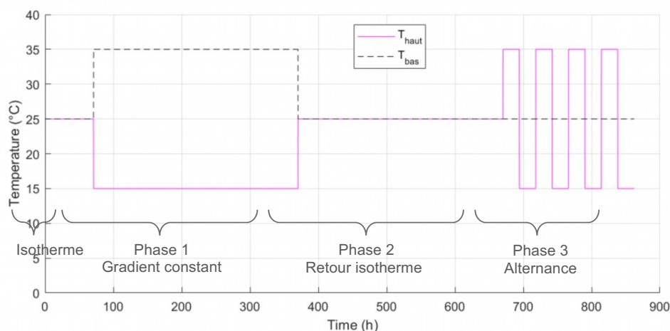
Fig. 2 : Consigne des températures appliquées sur les faces opposées de l'échantillon
