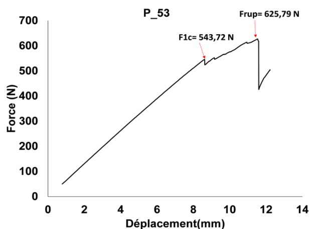
Fig. 4 : Courbe force-déplacement pour le Padouk - P53.
