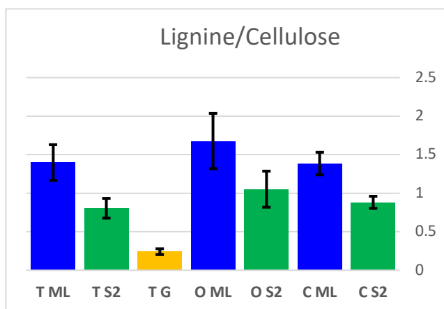
Fig. 5 : Ratio lignine/cellulose selon la couche de la paroi (Lamelle moyenne ML, paroi secondaire S2 et couche gélatineuse G) et la localisation dans la section de la tige (Tension T, Opposé O et Contrôle ou bois normal C)
