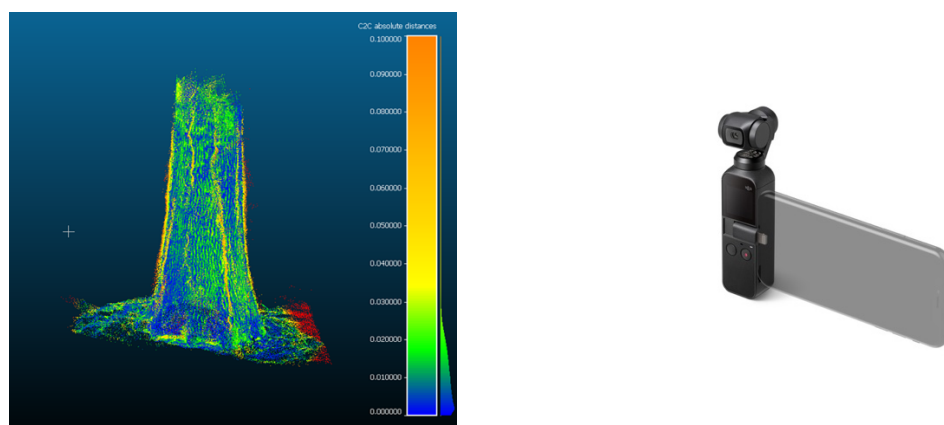
Fig. 2 : Illustration de premiers essais comparatifs entre données 3D provenant d'un Lidar terrestre et de la caméra stabilisée DJI-OSMO Pocket®.
