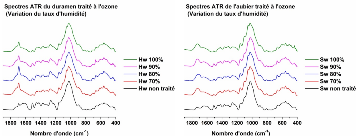
Fig. 2 : Spectres ATR des duramen (gauche) et aubier (droite) humidifiés après traitement à l'ozone
