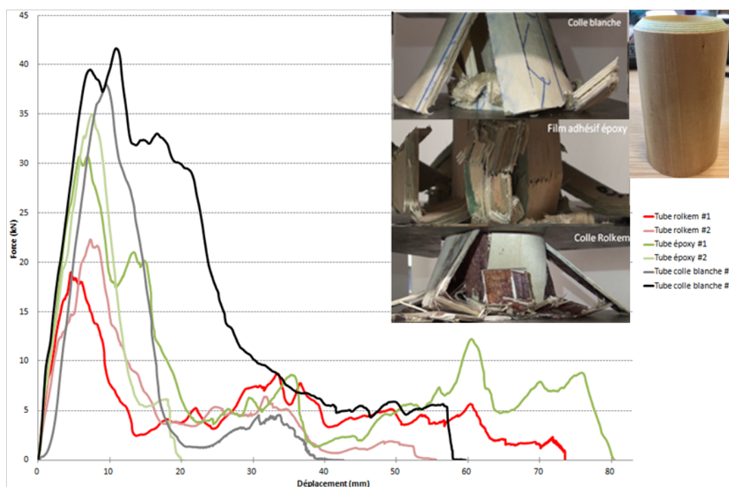
Fig. 3 : Influence des 3 types de colle sur les courbes force-déplacement pour des tubes bois
