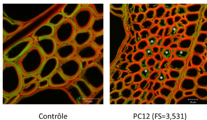
Fig4. Photographies après observations en CLSM (mode spectral) d'échantillons contrôle et explosés à la vapeur ( CS = 3,531 ). Le vert correspond à des zones pauvres en lignine et le rouge à des zones où cellulose et lignine sont présentes. Les astérisques indiquent les cellules où une « couche G like » est présente.
