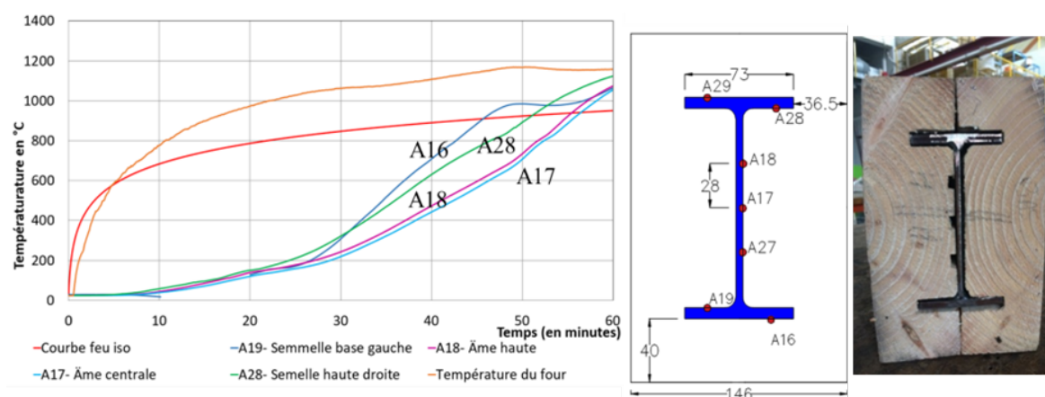
Fig. 5 : Température de l'acier d'une poutre protégée par du bois de pin
