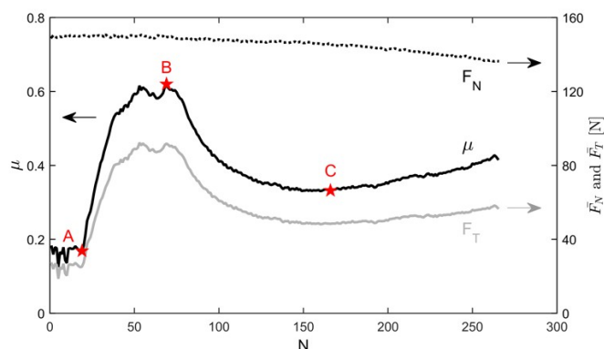
Fig.1 : Evolution de \mu_{moy} et F_N lors du soudage : jusqu'au A->évaporation de l'humidité dans le contact ; A->B : formation de débris d'usure sous forme de rouleaux ; B->C : formation d'un 3ème corps (phase optimale pour le soudage) ; après C : usure importante et dégradation du matériau
