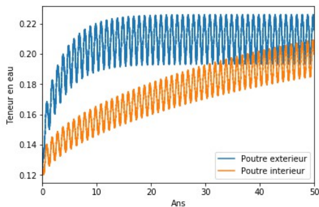
Fig. 4 : Evolution de teneur en eau moyenne par poutre sur 50 ans
