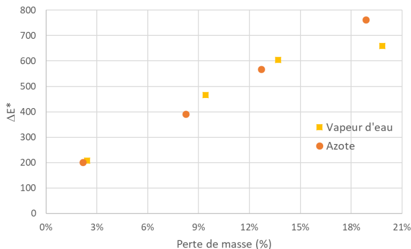
Fig. 3 : Evolution de la couleur du hêtre lors des traitements sous vapeur d'eau et sous azote.
