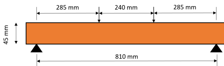
Figure 2 : Schéma de positionnement de l'éprouvette d'essai filles en flexion quatre points
