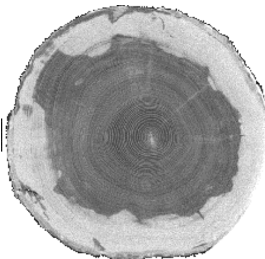
Fig. 2 : Image tomographique RX d'une section de grume d'épicéa
