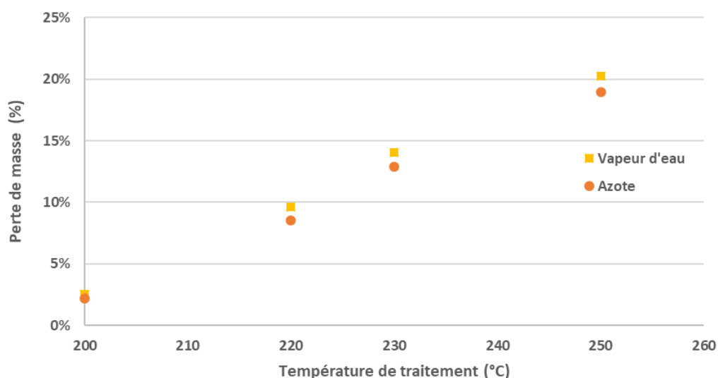
Fig. 2 : Influence de la température et de la composition de l'atmosphère sur la perte de masse lors du traitement thermique de bois de hêtre.
