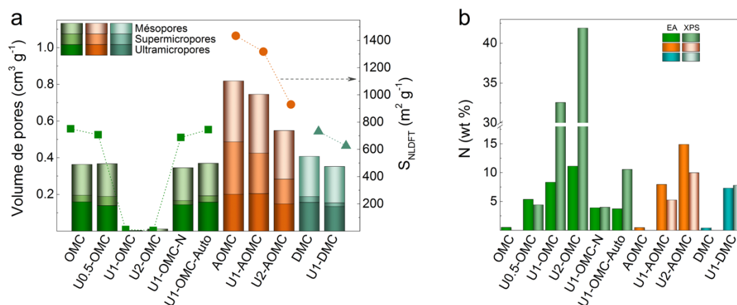
Fig. 1 : Propriétés physicochimiques des matériaux: (a) volume de pores (barres) et surface spécifique (S NLDFT , symboles) ; (b) teneur en N mesurée par EA et XPS.
