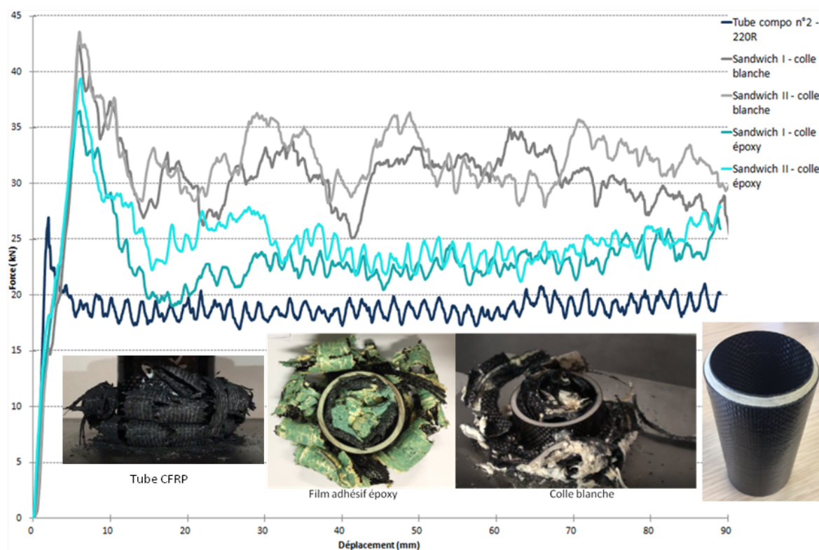
Fig. 4 : Influence de la colle sur les courbes force-déplacement des tubes sandwichs
