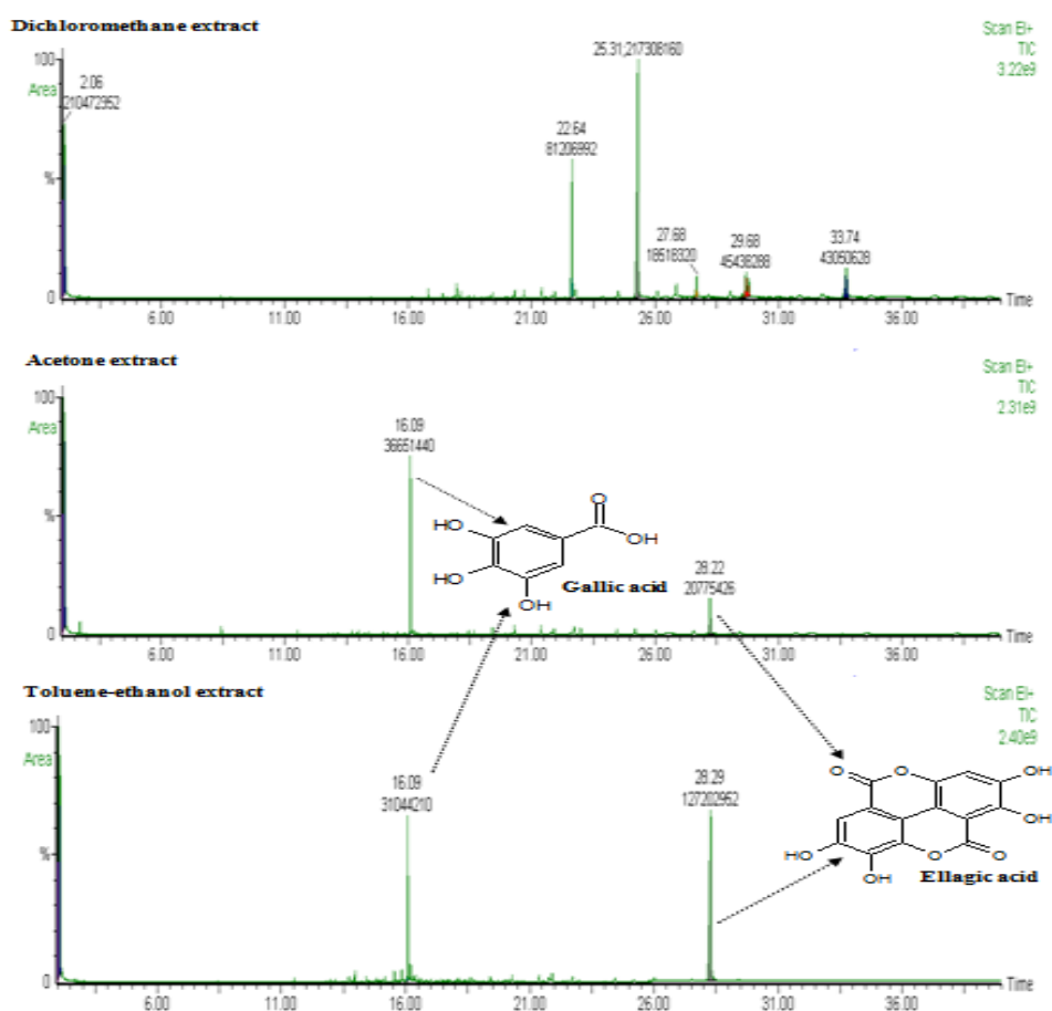
Fig.1 : Analyse GC/MS des différents extraits .
