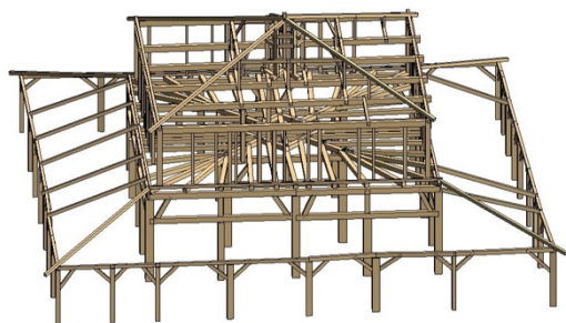
Fig. 3 : Aspect général de la structure de la halle
