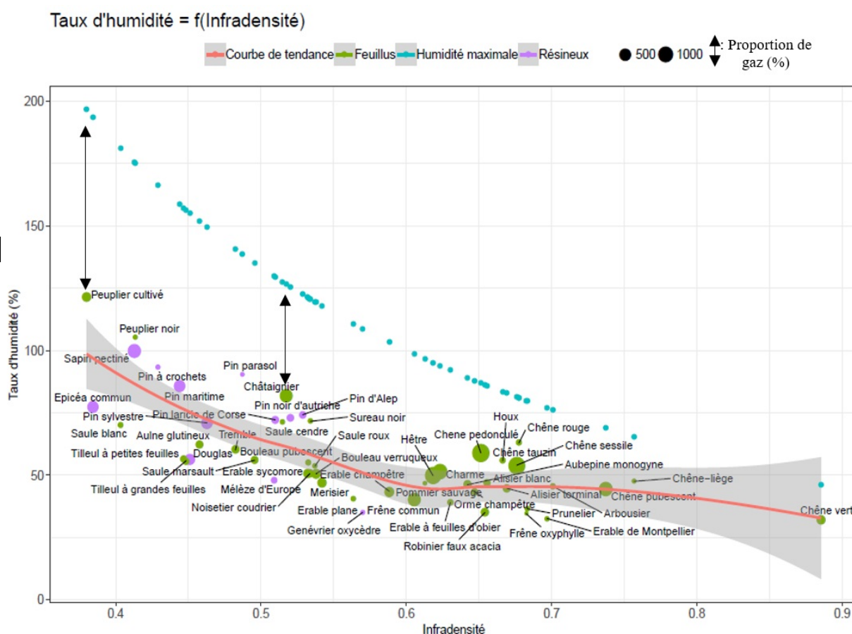
Fig 2 : Variation du taux d'humidité et de la proportion de gaz en fonction de l'infradensité
