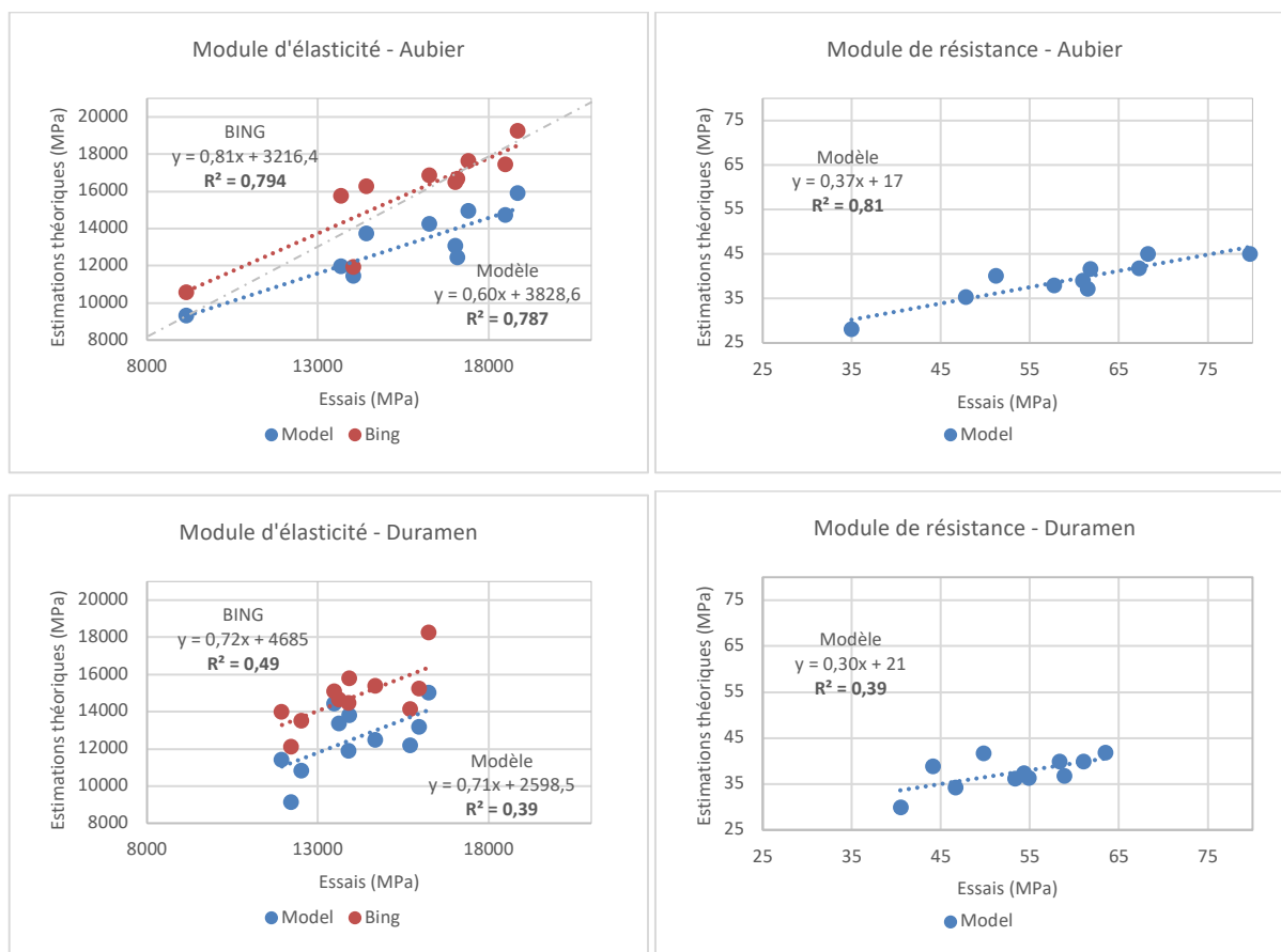
Fig. 3 : Comparaison essais mécaniques, essais vibratoires et modèle mécanique
