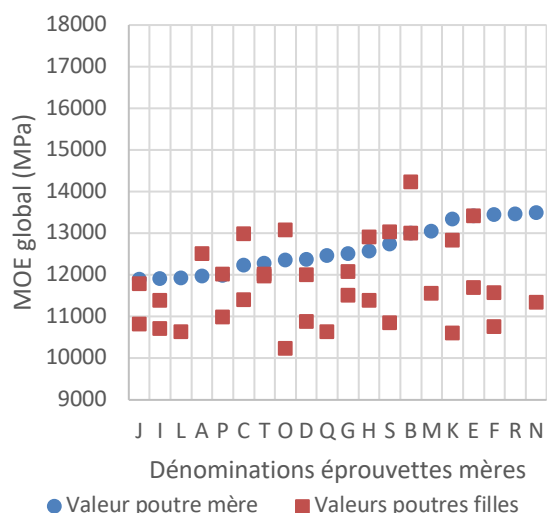
Figure 6 : Valeurs de modules élastiques globaux en flexion des corps d'éprouvettes parents et enfants
