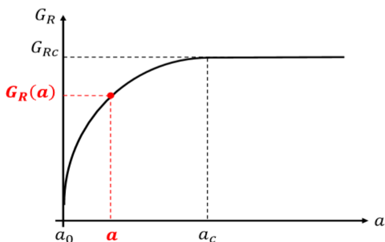
Fig. 3 : Courbe-R en mode pur (Morel 2007)
