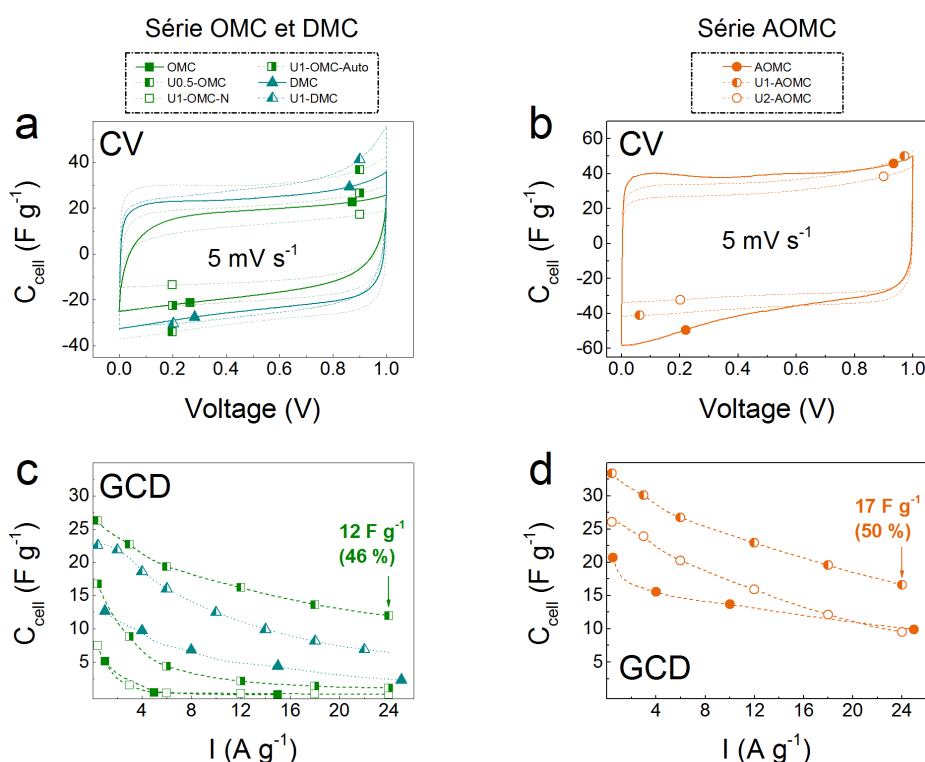
Fig. 2 : Performance électrochimique des matériaux : (a, b) courbes de CV à 5 \text{ mV s}^{-1} ; (c, d) capacitance ( C_{\text{cell}} ) en fonction du courant, calculé à partir des courbes de GCD.
