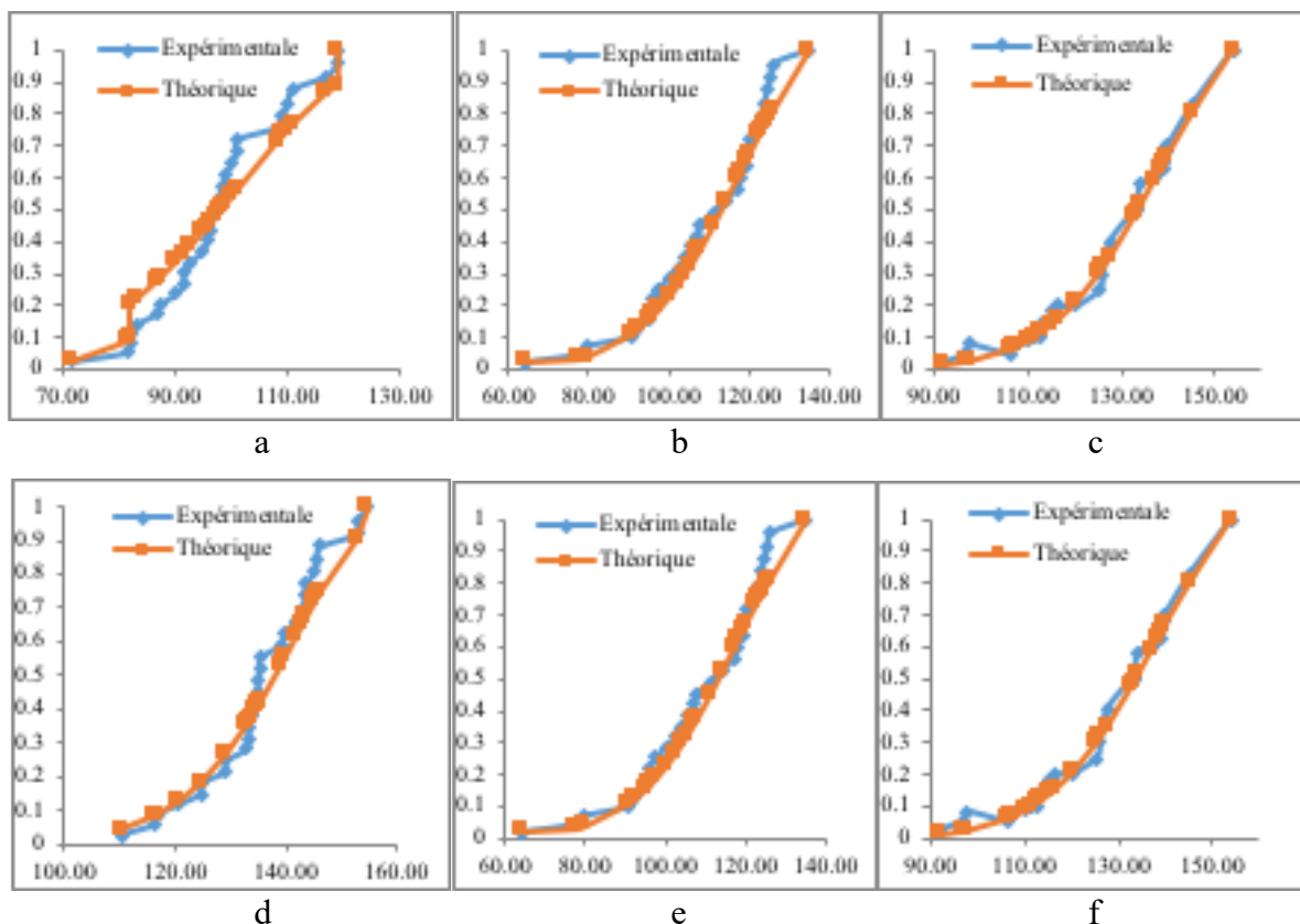
Fig. 5 : Distributions cumulées expérimentales et théoriques des contraintes à la rupture des échantillons de type I(a), type II(b), type III(c), type IV(d), type V(e), type VI(f)
