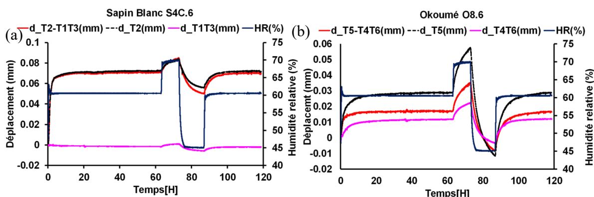
Fig. 6 : effet des variations de HR sur les baguettes (a) ; de Sapin Blanc (b) ; d'Okoumé
