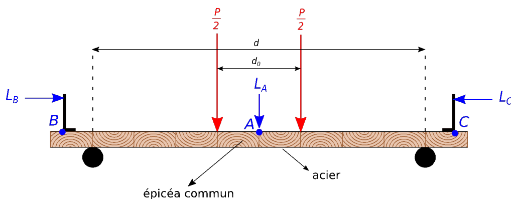
Fig. 1 : Essai de flexion 4-points sur une poutre sandwich
