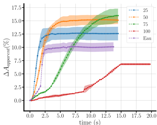
Fig. 3 : Evolution au cours du temps de la variation d'aire apparente des échantillons soumis à différents mélanges volumique eau / DMF.
