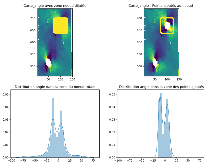
Fig. 1 : Étude de la zone de perturbation des fibres autour d'un nœud
