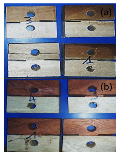
Fig. 4 : Mode de rupture des joints, (a) Ni-Oz, (b) Pdk-Oz
