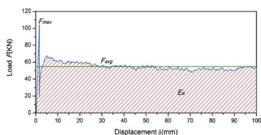
Fig. 2 : Courbe force-déplacement typique d'un tube circulaire composites en fibres de carbone/époxy (Sun et al., 2018)
