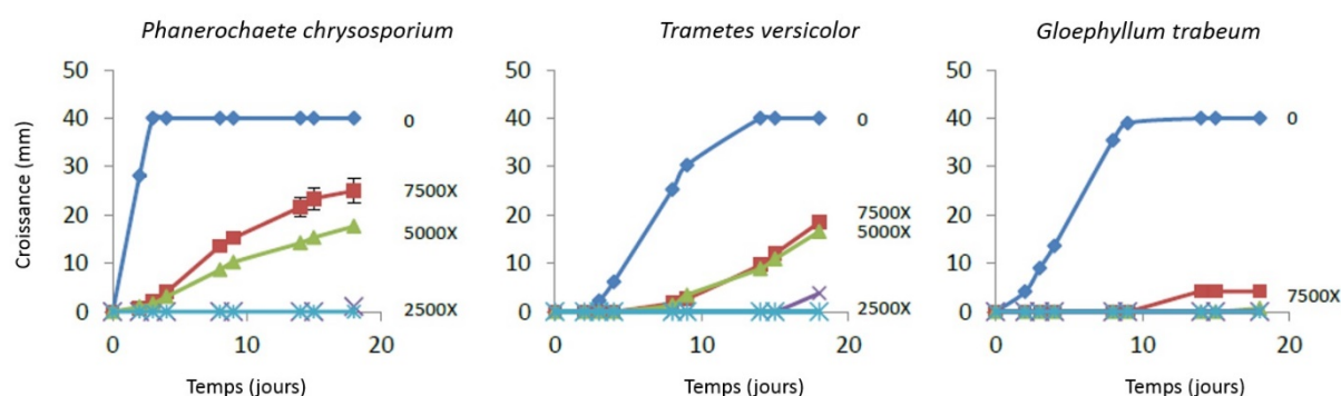
Fig.1 : Croissance de 3 souches fongiques en présence de Tanalith E3474 à différentes dilutions (de 2500 à 7500 X). La croissance est appréciée grâce à la mesure du diamètre de la colonie.
