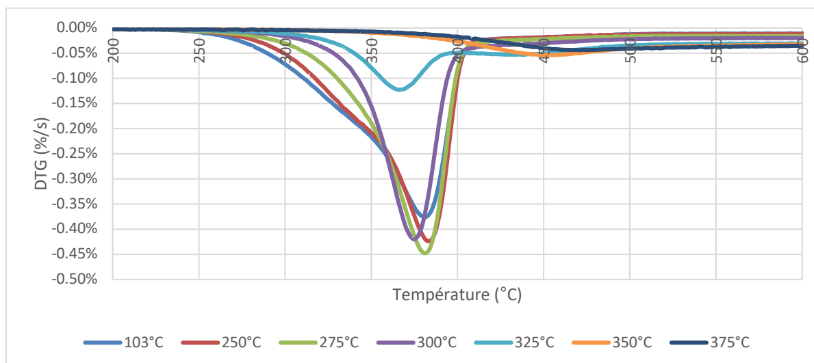
Fig. 6 : DTG du sapin. Valeurs pour un échantillon non traité (103°C) et pour différentes températures de traitement.
