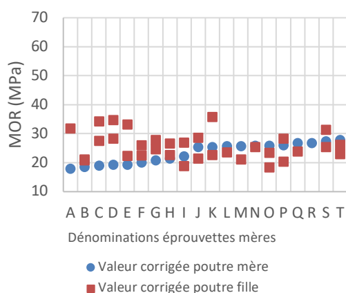
Figure 5 : Valeurs corrigées de contraintes de rupture en flexion (équation 1) des corps d'épreuves mères et filles
