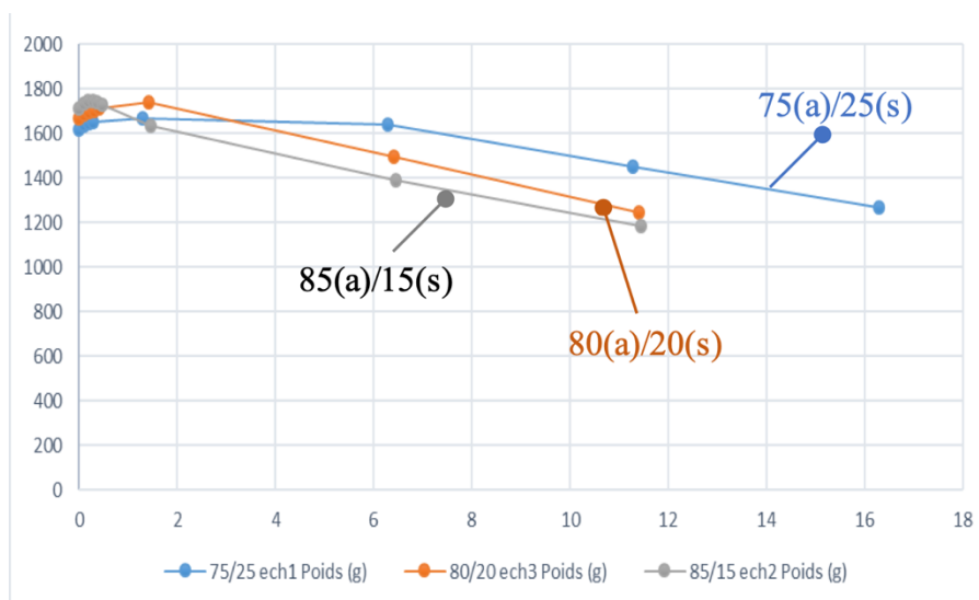
Fig. 3 : Variation du poids de l'échantillon en fonction du temps pour un pourcentage argile / sciures : (a) 75a/25s ; (b) 80a/20s ; (c) 85a/15s.
