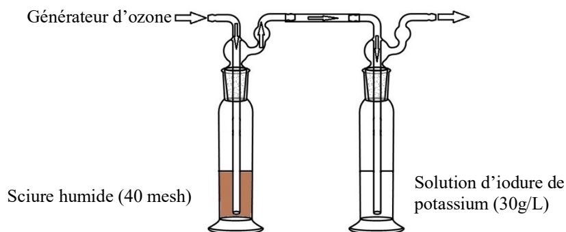
Fig. 1 : Montage de traitement à l'ozone
