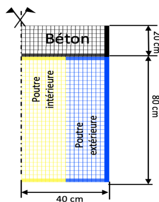
Fig. 2 : Maillage d'une demi-section transversale
