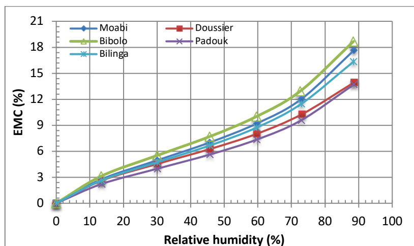
Fig. 1 : Isotherme d'adsorption à 35°C
