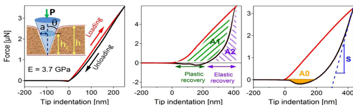
Fig. 2 : Extraction des différentes propriétés mécaniques à partir des courbes force-déplacement acquises par nano-indentation.
