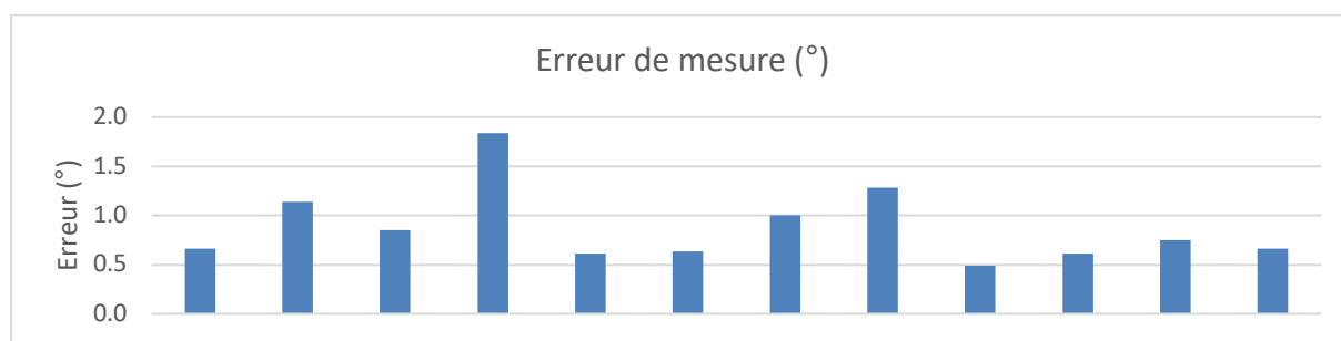
Fig. 3 : Erreur de mesure de l'orientation des fibres en fonction des plans LR et LT et des essences
