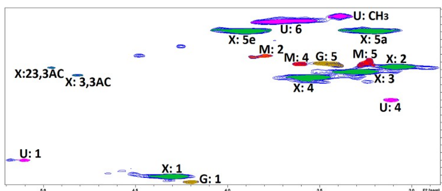
Fig. 3: RMN 2D HSQC des hémicelluloses extraites au DMSO :
