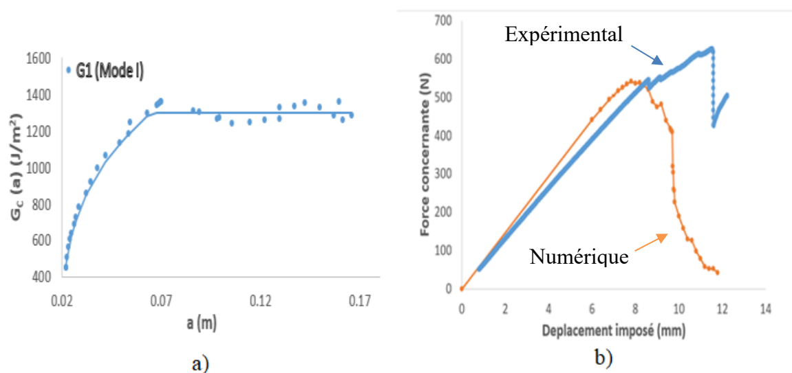
Fig. 5: Confrontation numérique expérimental : (a) Courbe-R en mode I de l'éprouvette P53 ; (b) Courbes Force-Déplacement de l'éprouvette P53
