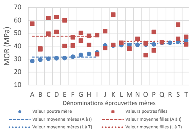
Figure 4 : Valeurs de contraintes de rupture en flexion des corps d'épreuves parents et enfants
