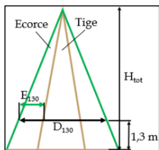
Fig. 3 : Schéma de modélisation d'une tige modélisée par une suite de troncs de cônes
