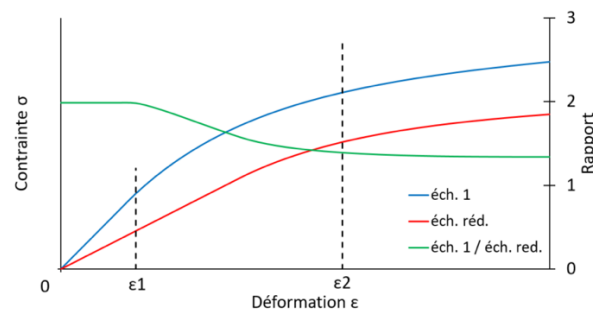
Fig. 3: Lois de comportement non linéaires
