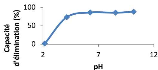
Fig. 2: Effet du pH sur l'adsorption du bleu de méthylène (à 100ppm) par des coques broyées de Lophira à 25^{\circ}\text{C} , après 180mn de contact
