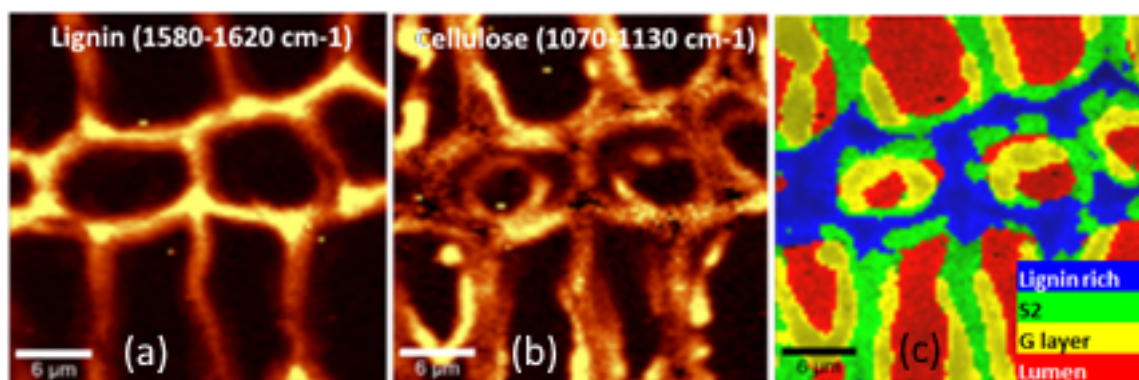
Figure 4 : Cartes obtenues par spectroscopie Raman sur du bois de tension. (a) intégration du signal dans la gamme 1580\text{-}1620\text{cm}^{-1} caractéristique de la lignine, (b) intégration du signal dans la gamme 1070\text{-}1130\text{cm}^{-1} caractéristique de la cellulose, (c) clusters obtenus par partition en k-moyennes ( k = 4 ).
