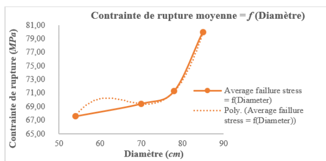
Fig. 4 : Courbe d'évolution des différentes contraintes moyennes de rupture
