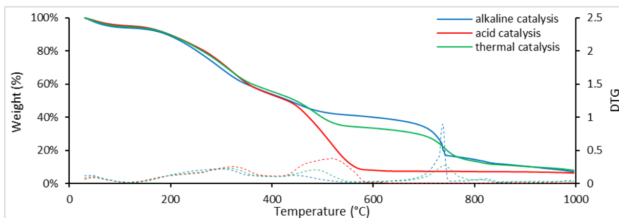
Fig. 1. Analyse thermogravimétrique.
