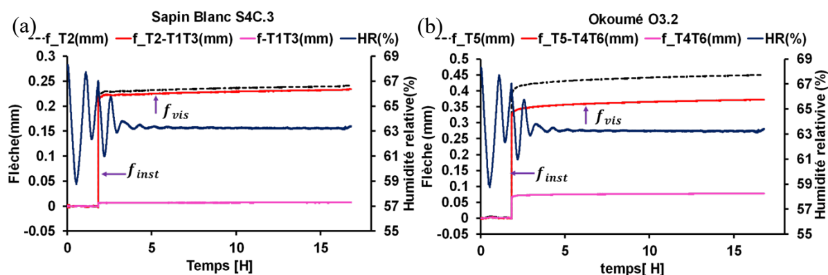
Fig. 7 : mise en évidence du comportement viscoélastique des baguettes (a) : Sapin Blanc (b) : Okoumé
