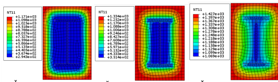
Fig. 7 : Modèle 2D d'une poutre mixte bois acier (température à 15, 30, 60 minutes en K)
