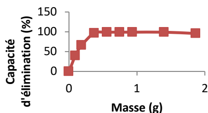
Fig. 1: Effet de la masse de coques broyées de Lophira sur l'élimination du bleu de méthylène (100ppm) à 25^{\circ}\text{C} après 1200mn de contact
