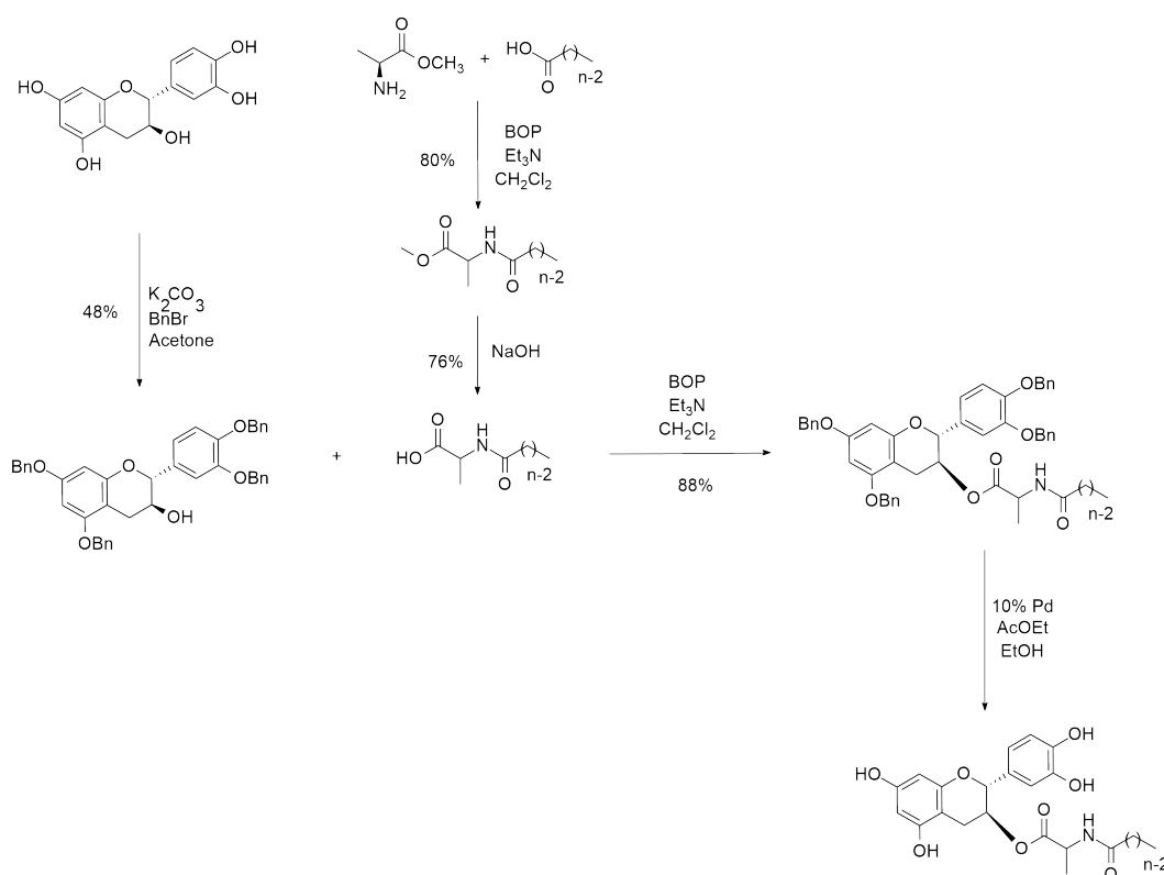
Fig. 2 : Synthèse du composé tri-modulaire. n=10
