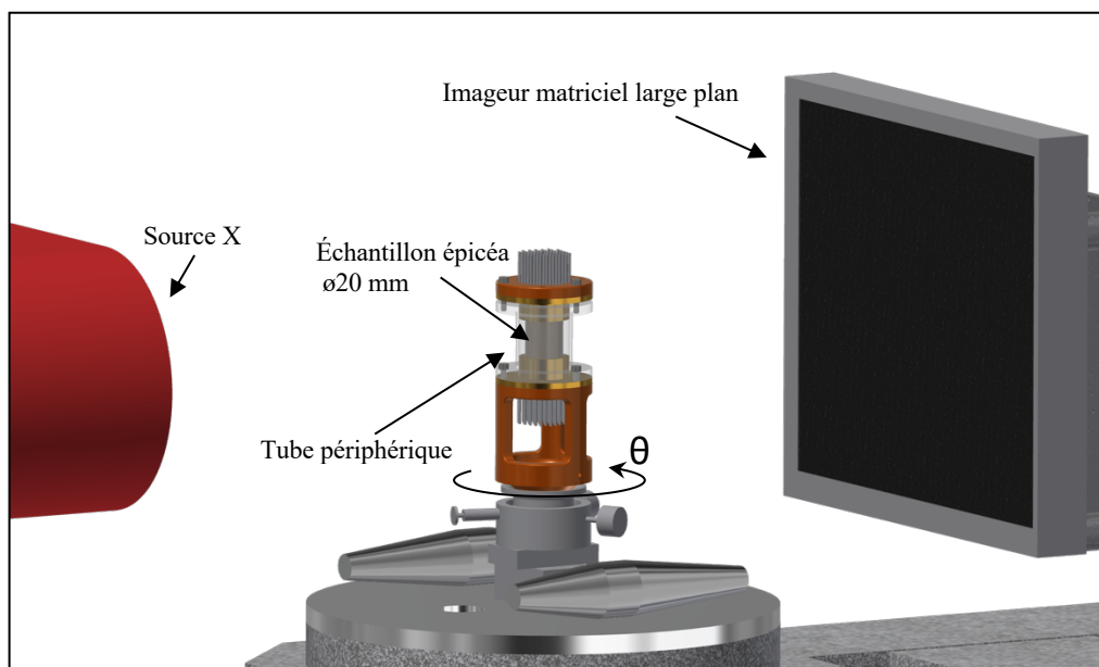
Fig. 1 : Schéma du dispositif expérimental de thermo-diffusion 3D
