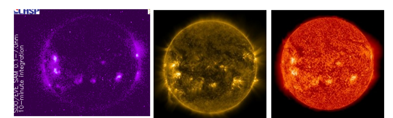
Couronne 10 6 K, Zone de Transition 10 5 K, photosphère 6000 K
