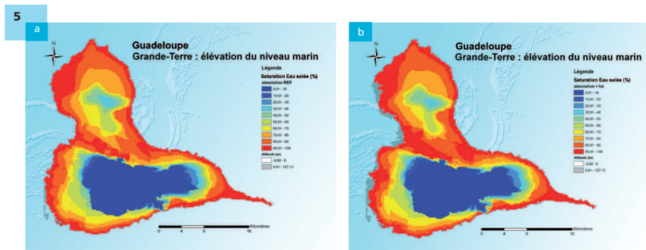
Figure 5. Saturation de l'aquifère en eau salée pour la situation de référence et pour une élévation du niveau marin de 1 m NGG (niveau général guadeloupéen) en Guadeloupe. La figure (a) montre la situation actuelle (situation REF), la figure (b) montre la simulation avec une élévation du niveau marin de 1 m NGG
