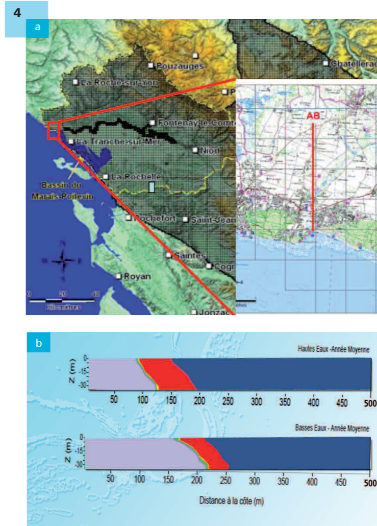
Figure 4. Avancée du biseau salé pour différents scénarios de remontée océanique sur un transect du Marais Poitevin (Le front équivalent à une concentration de 100 mg.L -1 de chlorures).
