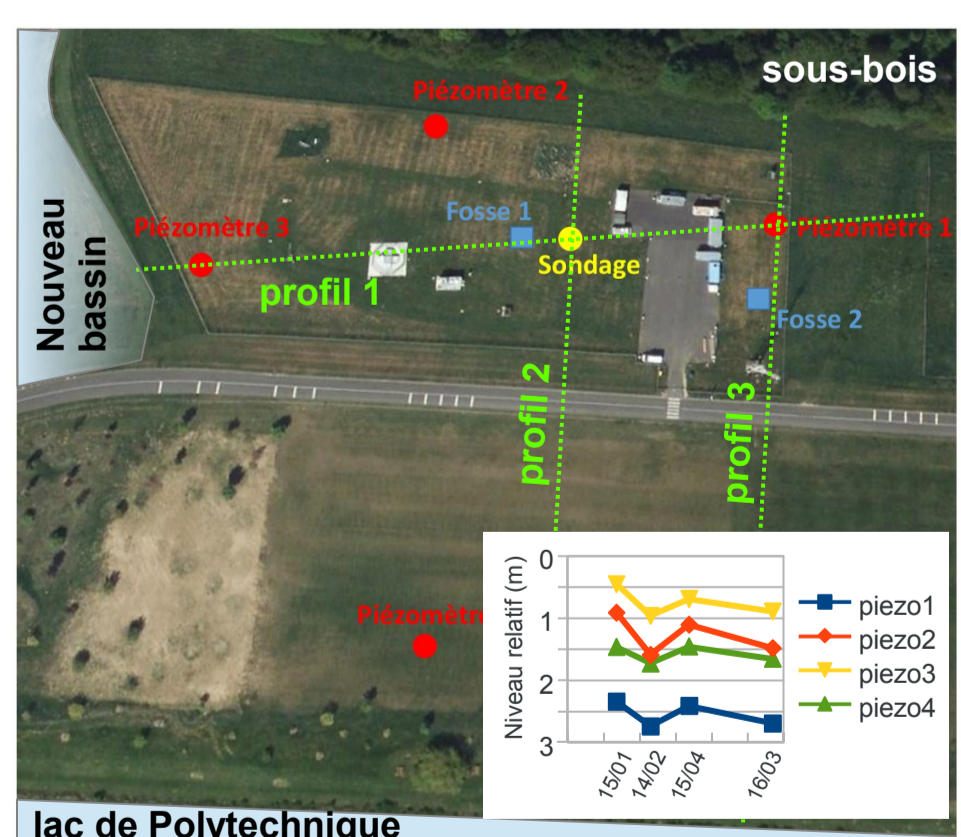
Figure 4 : Nouveaux piézomètres en croix et sondage à l'emplacement de la première fosse TDR. (En incrustation) : les premiers relevés de profondeur du niveau saturé montrent une évolution synchrone mais des valeurs absolues significativement différentes en partie liées à la topographie (CEREMA 2015).
