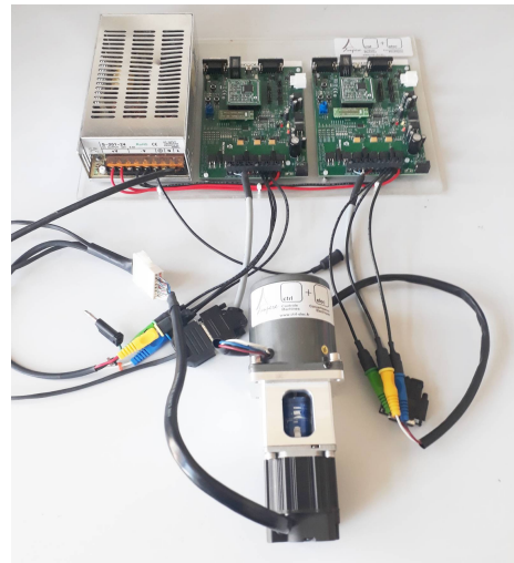
Fig. 4. AC motors
