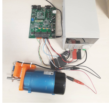
Fig. 3. DC motor
