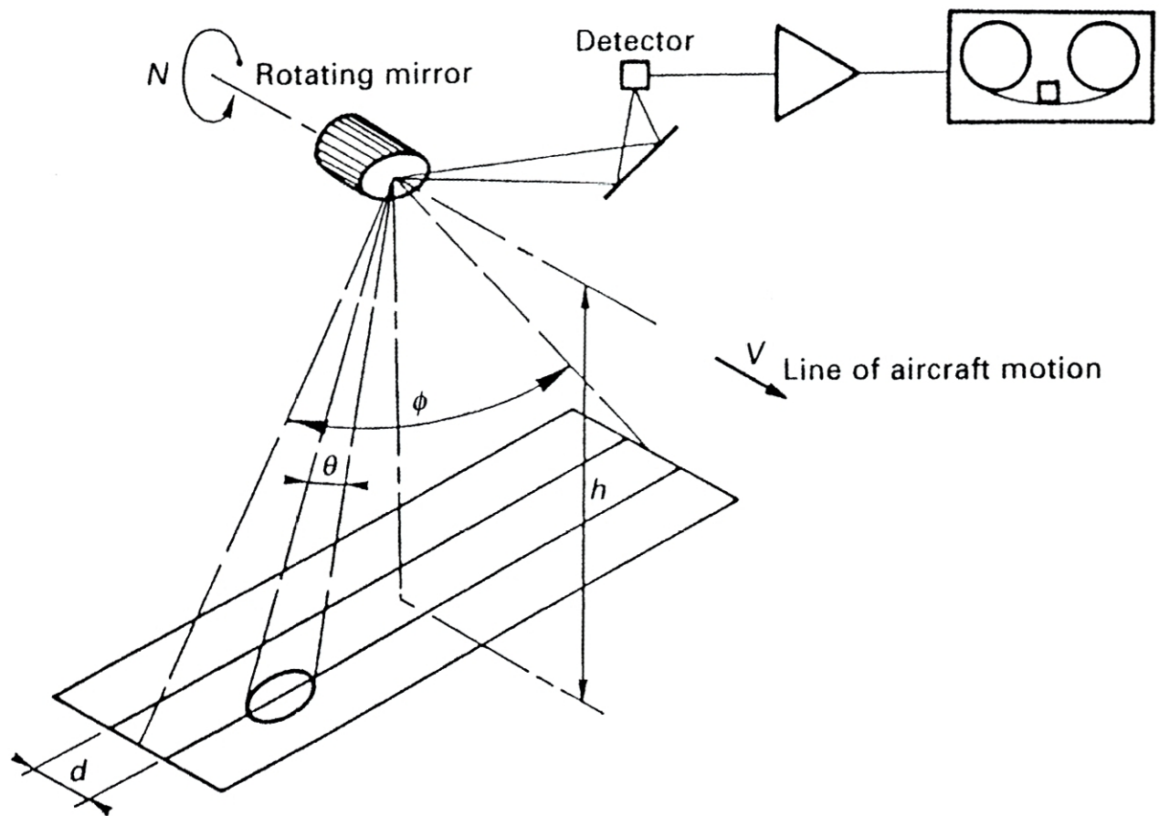
Fig. 1 : un radiomètre aéroporté. An air borne radiometer.
