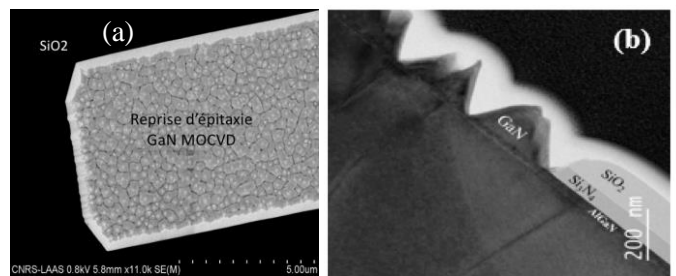
Fig. 9 : Images MEB de la reprise d'épitaxie du GaN par MOCVD après gravure chlorée de l'AlGaIn pendant 25 s : (a) vue de dessus d'une ouverture de grille de 6μm, (b) vue en coupe.
