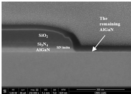
Fig. 7 : Image FIB après gravure RIE de l'AlGaIn par Cl 2 en 35 s.
