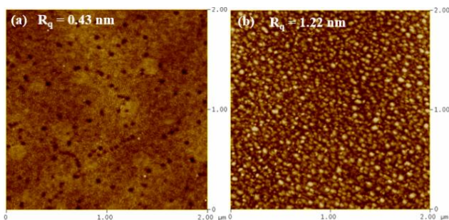
Fig.8 : Images AFM de l'AlGaIn : (a) avant gravure, (b) après gravure RIE par Cl 2 pendant 25 s (puissance RF = 60 W, pression = 5 mTorr and Cl 2 flow = 10 sccm).
