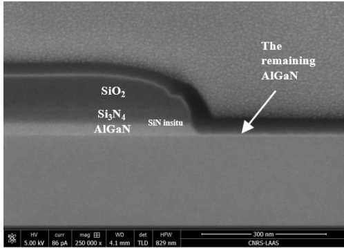
Fig. 7 : Image FIB après gravure RIE de l'AlGaN par Cl 2 en 35 s.
