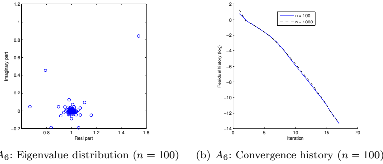
Fig. 5 Matrix A_6 .
