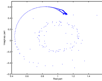
(d) Eigenvalue distribution.
