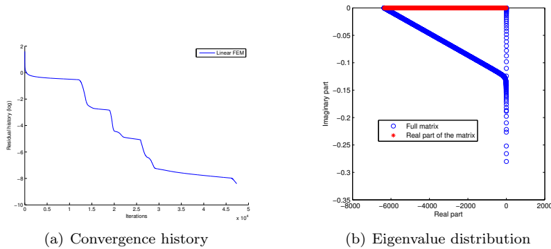
Fig. 7 Matrix (S_h - k^2 M_h - ikB_h) .
