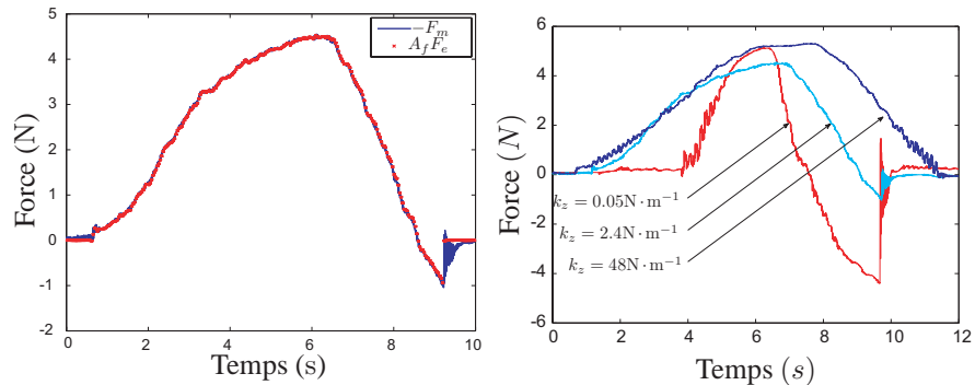
(a) poutre utilisée : k_z = 2,4 \text{ N} \cdot \text{m}^{-1} ( A_d = 0,05 \cdot 10^6 , A_f = 6 \cdot 10^6 )
