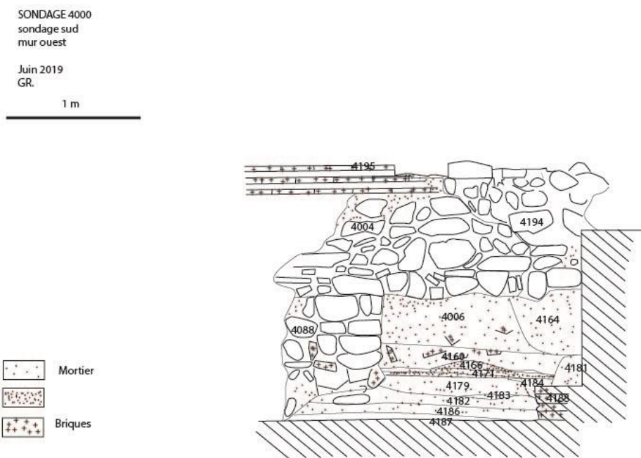
Fig. 22: élévation des murs MR 4004 et 4194 (RAFAD 2019)
