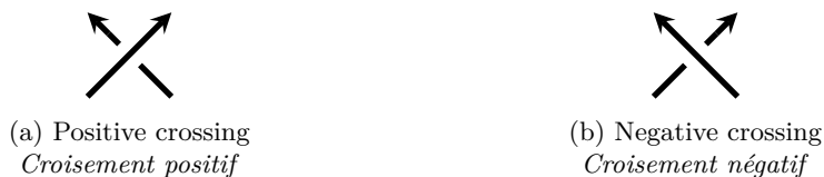
Figure 2: Each crossing of an oriented knot can be identified to one of Figure 2a or 2b. Tout croisement d'un nœud orienté peut être identifié à l'une des figures 2a ou 2b.
