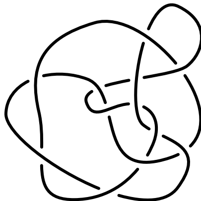
Figure 1 – A representation of \gamma , a 3-trivial prime knot with 12 crossings [2, knot 12n659]. Une représentation de \gamma , un noeud 3-trivial premier avec 12 croisements [2, knot 12n659].
