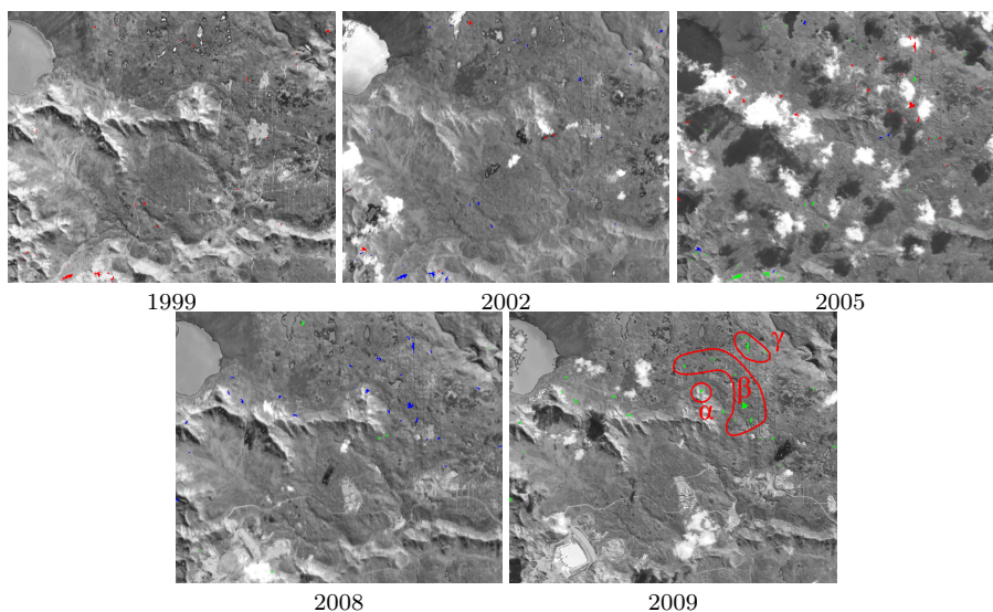
Fig. 13: Pattern NDVI_2 \xrightarrow{57} NDVI_3 \xrightarrow{58} NDVI_4
