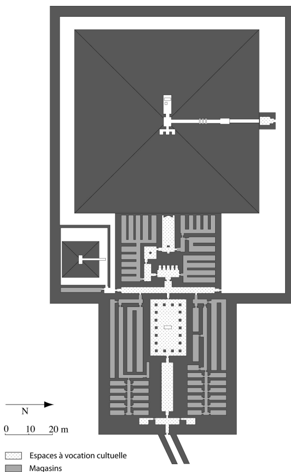
Figure 1. Plan du temple haut du pharaon Pépy I er (© Mafs)
