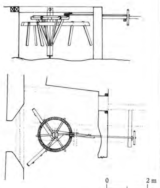
Saint-Max (54), Champenoux, maison, manège à chevaux, plan, élévation et vue perspective (relevé schématique).
