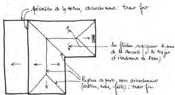
Croquis de plan masse.
