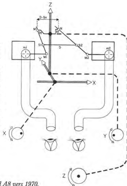
Restituteur analogique Wild A8 vers 1970.
