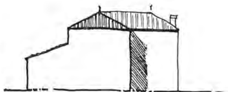
Croquis en plan et élévation indiquant les codes de représentations des toitures.
