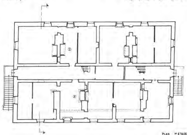
Bains-les-Bains (88), manufacture royale de ferblanterie, plans et coupe transversale (relevé manuel).
