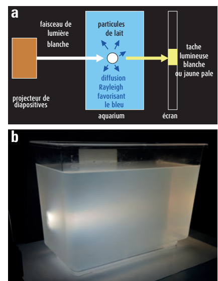
Figure 5. a) Schéma du dispositif expérimental de la troisième expérience. b) Photographie du bac traversé par le faisceau lumineux. On peut voir la coloration bleutée de l'eau dans la moitié du récipient près de la face d'entrée du faisceau. L'eau devient jaune dans la partie droite du récipient.
