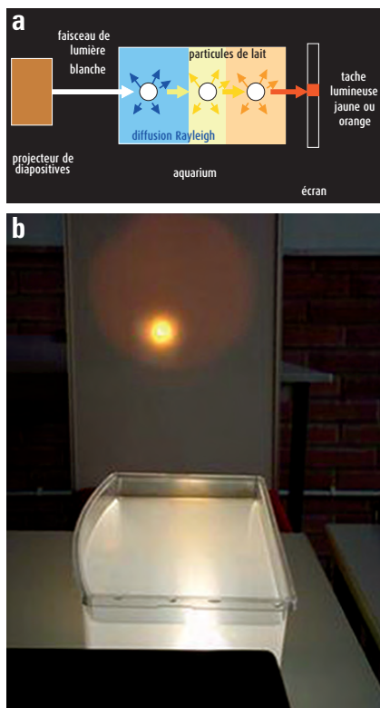
Figure 6. a) Schéma du dispositif expérimental de la quatrième expérience. Le faisceau traversant le bac permet d'illustrer que le ciel devient orangé au lever ou au coucher de soleil. b) Photographie du bac traversé par le faisceau lumineux qui devient orangé. On voit la tache orangée sur l'écran.
