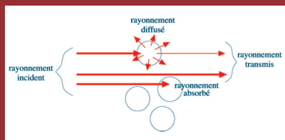
Figure E1. Schéma très simplifié des principaux mécanismes que peut subir le rayonnement lumineux en rencontrant des molécules ou particules : transmission, absorption, diffusion.
