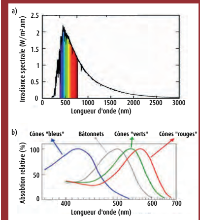
Figure E3. a) Spectre de la lumière solaire en fonction de la longueur d'onde. La lumière visible correspond à des longueurs d'onde comprises entre 380 et 750 nm. b) Spectre de réponse des photorécepteurs de l'œil humain, d'après Bowmaker et Dartnall (1980).
