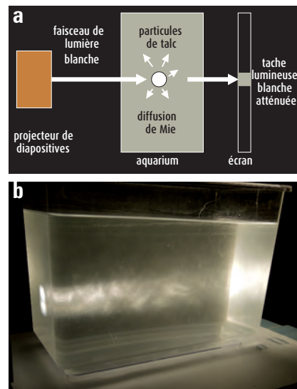
Figure 3. a) Schéma du dispositif expérimental de la deuxième expérience. b) Photographie du bac traversé par le faisceau lumineux.
