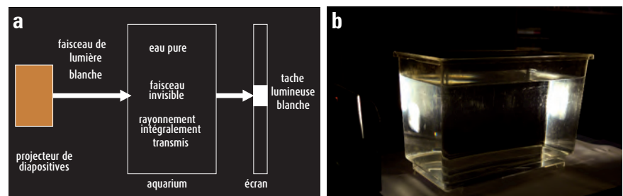
Figure 1. a) Schéma du dispositif expérimental de la première expérience. b) Photographie du bac traversé par le faisceau lumineux.
