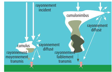
Figure 4. Schéma expliquant pourquoi les nuages sont blancs ou gris pour un observateur au sol. Si l'observateur reçoit surtout la lumière diffusée, blanche, il voit le nuage blanc. Si l'observateur ne reçoit qu'une petite partie de la lumière incidente, à cause de la réflexion, diffusion ou absorption, il voit le nuage ou les parties de nuage grises, d'autant plus foncées qu'il reçoit moins de lumière incidente.
