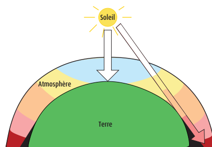
Figure 7. Schéma montrant pourquoi le ciel est bleu à midi et devient orangé au lever ou au coucher de soleil.
