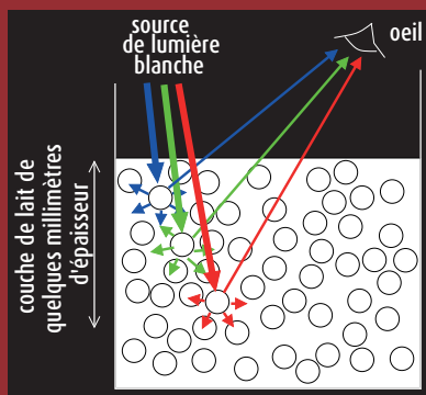
Figure E2. Schéma montrant pourquoi l'œil humain voit le verre de lait blanc, alors que les particules de lait diffusent préférentiellement la lumière bleue.
