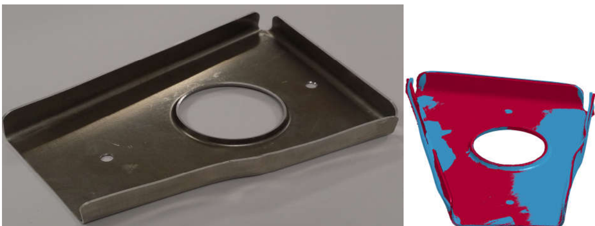
Figure 8 : formage magnétique d'une pièce échelle 1 / comparaison simulation avec le logiciel LS DYNA (en bleu) et pièce réelle (en rouge)
