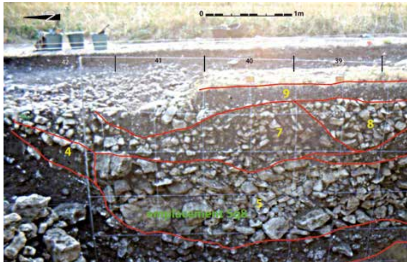
Fig. 3. Coupe de la diaclase recreusée avec son comblement. La couche 5 est concernée par les dépôts osseux humains (cl. et DAO J.-M. Large).
