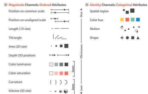
Fig. 3-3. Munzner’s guideline [4]
