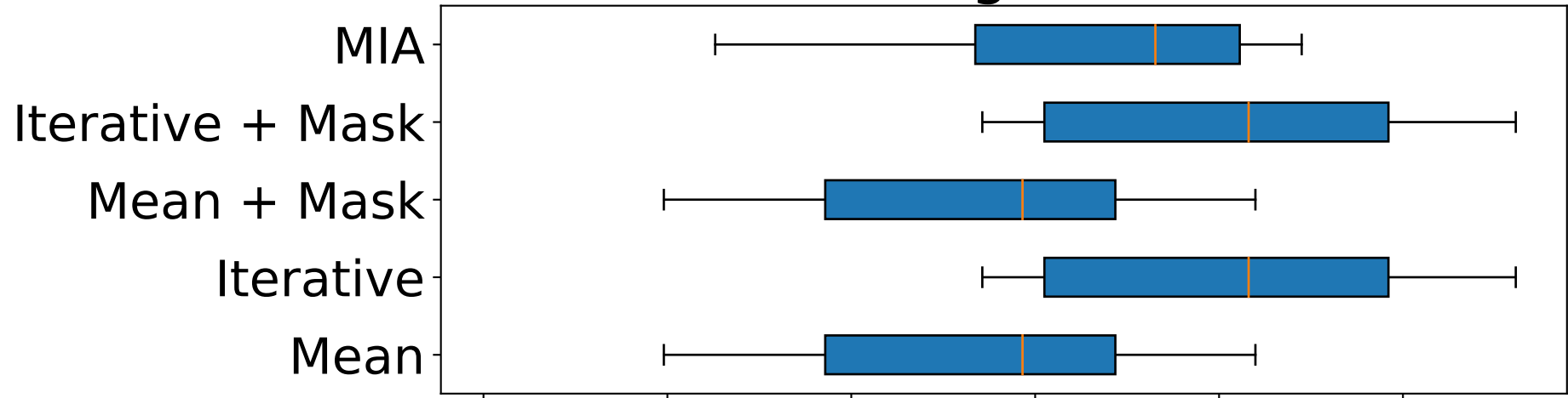
LinReg MNAR
