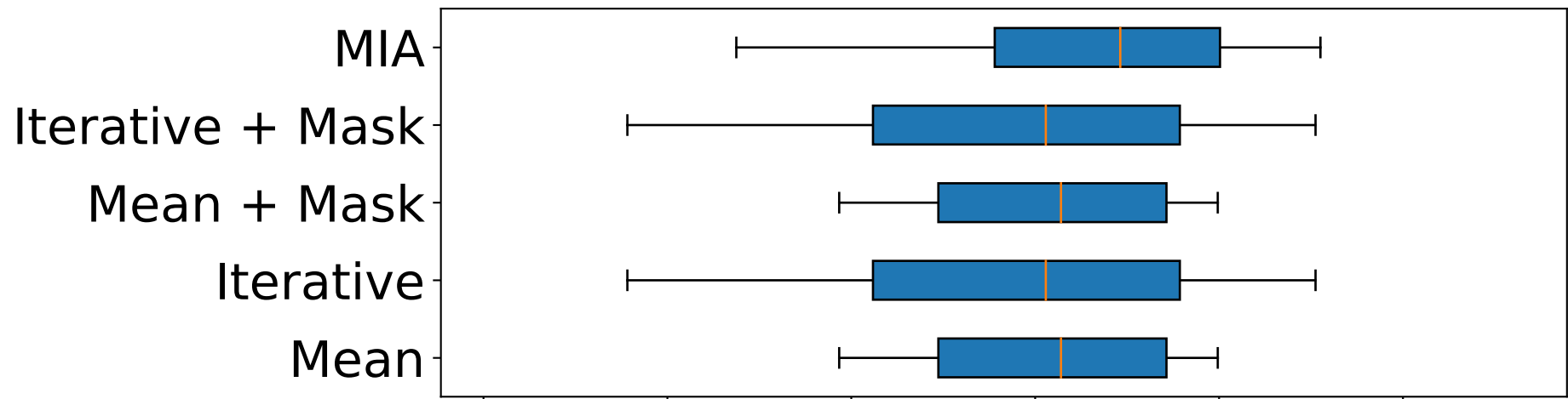
HGBoost MNAR
