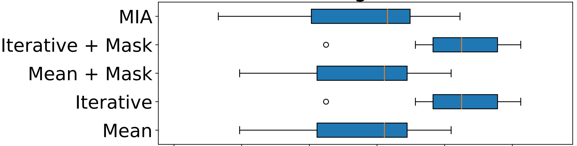
LinReg MCAR
