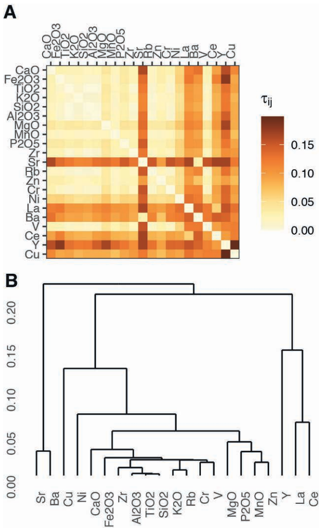
Figure 4 : Nicolas FRERE BEAU et al. , Analyse de données de composition et identification des altérations géochimiques des matériaux céramiques : le cas des productions d'un atelier ibérique (p. 40)
