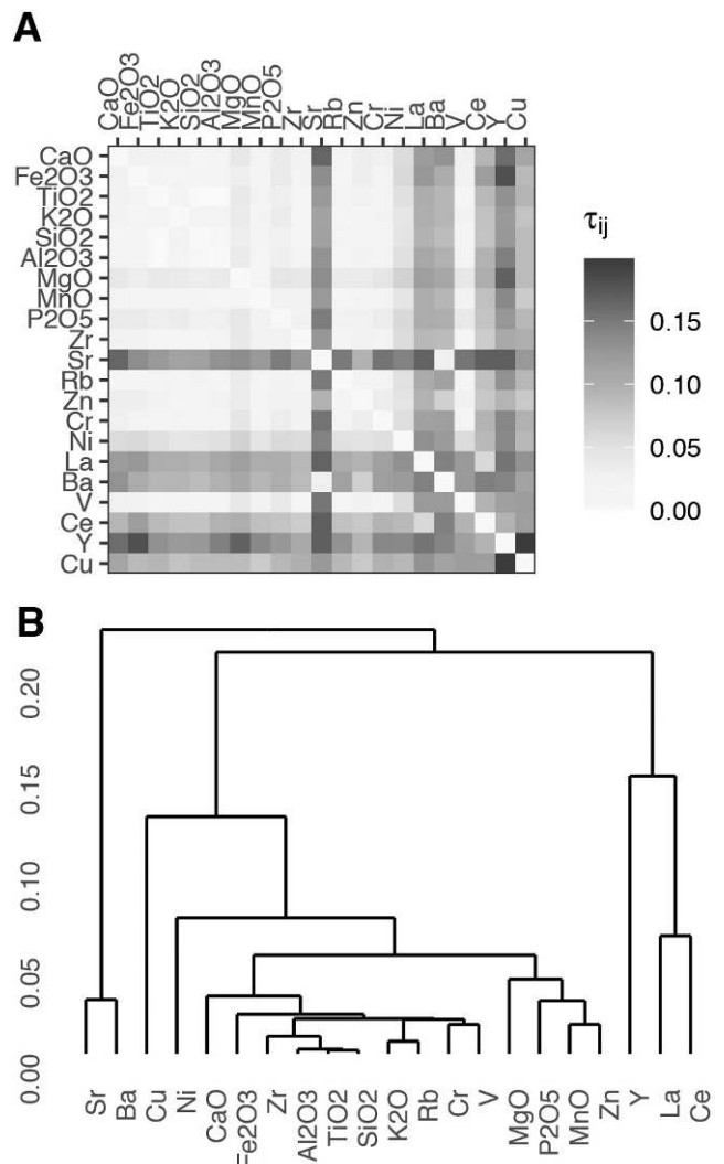
Figure 4 : (Voir planche couleur V) (A) matrice de variation de l'ensemble du corpus (terres crues et céramiques) ; (B) classification des variables obtenue par la méthode d'agglomération de Ward à partir de la matrice de variation utilisée comme matrice de distance. Figure 4: (See colour plate V) (A) variation matrix of the whole dataset (ceramics and unfired sherds) ; (B) hierarchical classification of the variables using the variation matrix as a distance matrix (Ward agglomeration method).
