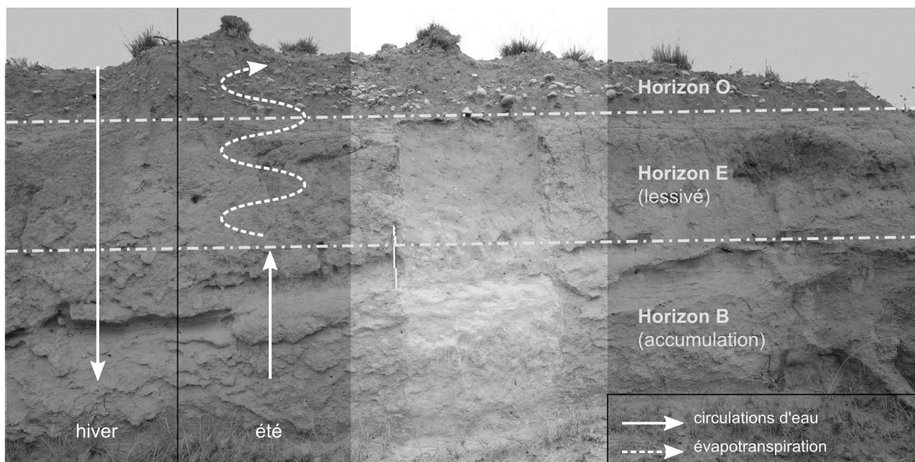
Figure 7 : Profil pédologique typique d'un calcisol à proximité du site du Mas de Moreno (Foz-Calanda, Teruel, Espagne). Au cours de l'hiver, les précipitations entraînent le lessivage des horizons supérieurs. À l'inverse, au cours de l'été, l'importante évapotranspiration entraîne la remontée de sels, qui s'accumulent dans l'horizon B. L'horizon d'accumulation, où se concentrent éléments alcalins et alcalino-terreux entraînant la précipitation de sels, est identifiable par sa teinte blanchâtre.
