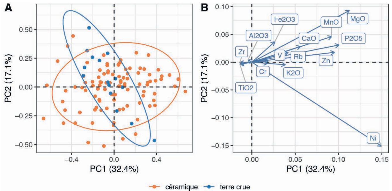
Figure 10 : Nicolas FREREBEAU et al. , Analyse de données de composition et identification des altérations géochimiques des matériaux céramiques : le cas des productions d'un atelier ibérique (p. 46)
