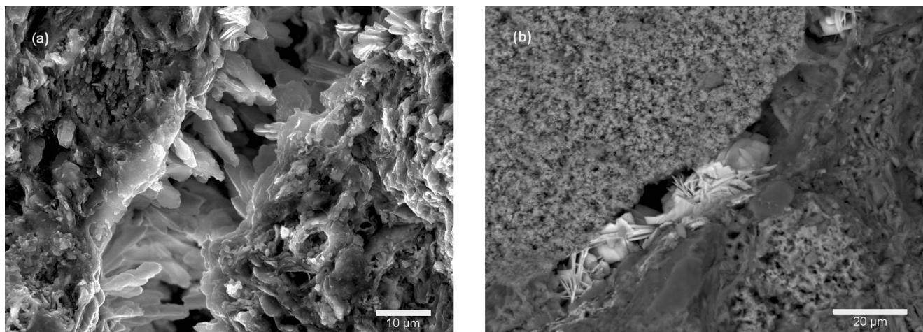
Figure 6 : Cristallisations secondaires dans les pores des matrices céramiques (microscopie électronique à balayage). (A) Cristaux de carbonates de calcium (calcite). Échantillon BDX15033, image en électrons secondaires. (B) Cristaux de sulfates de baryum (barytine). Échantillon BDX15034, image en électrons rétrodiffusés (les cristaux sont bien mis en évidence par le contraste chimique et apparaissent plus clairs).
