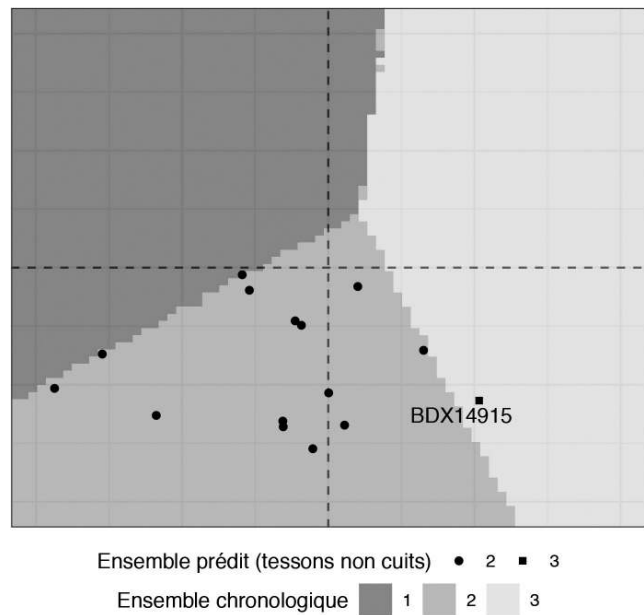
Figure 9 : (Voir planche couleur VI) Résultats de la LDA des compositions de l'ensemble du corpus après transformation (ILR). Le modèle a été construit à partir du corpus des céramiques afin de prédire l'appartenance des tessons non cuits à un ensemble chronologique sur la base de leurs compositions. Une approximation des frontières de décision de la LDA est également figurée, elle a été réalisée à l'aide d'une recherche par grille.
