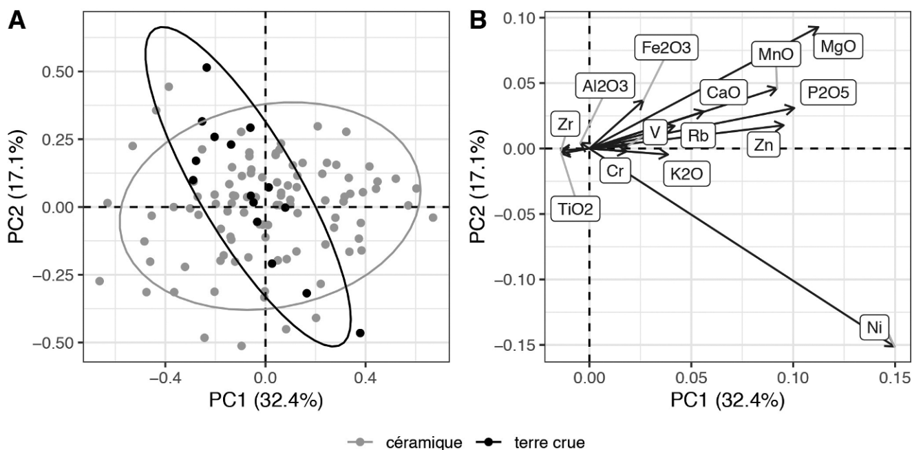
Figure 10 : (Voir planche couleur VI) Résultats de l'ACP centrée et non réduite des compositions de l'ensemble du corpus après transformation (ALR) en utilisant SiO_2 comme dénominateur. (A) projection du nuage des individus; (B) projection des variables.
