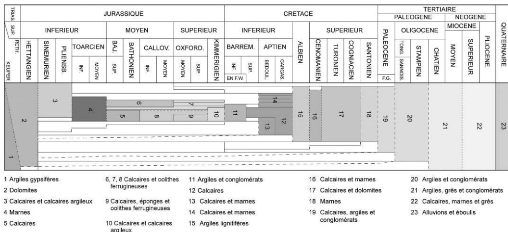
Figure 1 : (Voir planche couleur IV) Extrait de la carte géologique de l'Espagne au 1:50 000, feuille n° 494 (pour une légende détaillée, voir IGME, 1974) © Instituto Geológico y Minero de España.
