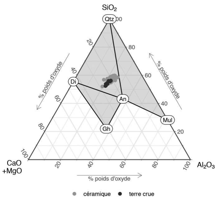
Figure 3 : (Voir planche couleur V) Compositions élémentaires des terres crues et des céramiques dans le système ternaire (CaO+MgO)-Al_2O_3-SiO_2 . Les trois domaines illustrés correspondent à la classification proposée par Noll (1991 ; de bas en haut et de gauche à droite : céramiques très calciques, céramiques calciques, peu calciques ; Di : diopside ; An : anorthite ; Gh : géhénite ; Mul : mullite ; Qtz : quartz).
