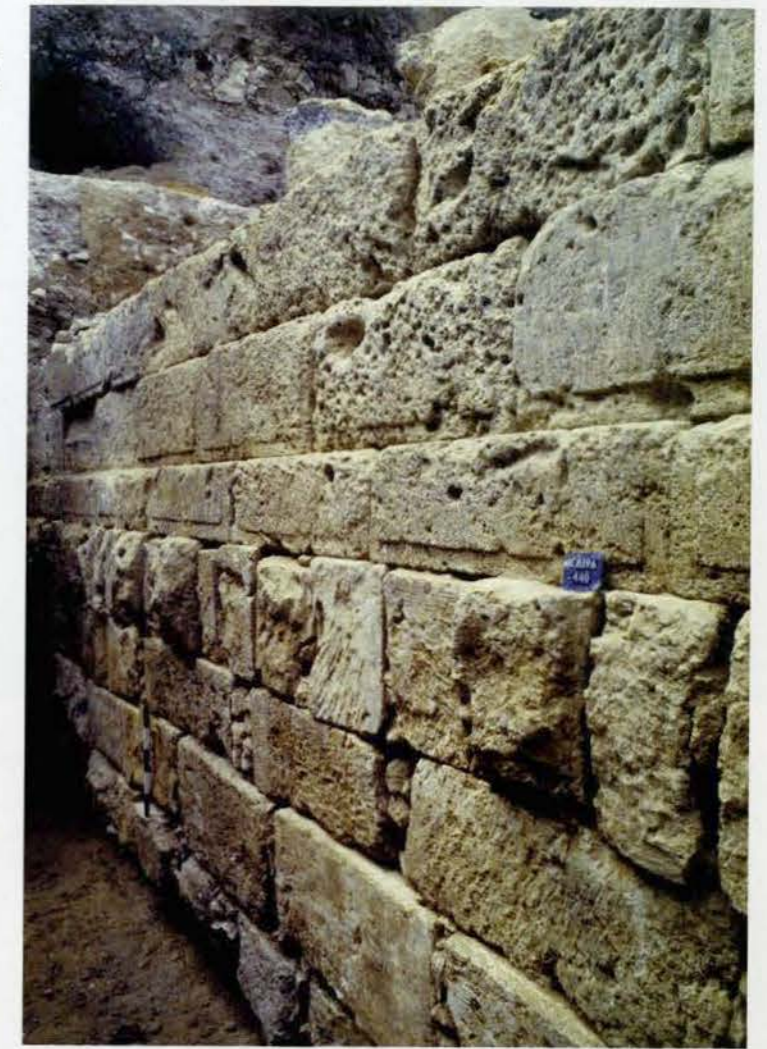
Chantier du Cricket Ground, mur de terrasse installé sur le rocher, bâti en blocs calcaires, et les trois premières assises du mur de façade de la maison (époque hellénistique). © CEALex/CNRS
