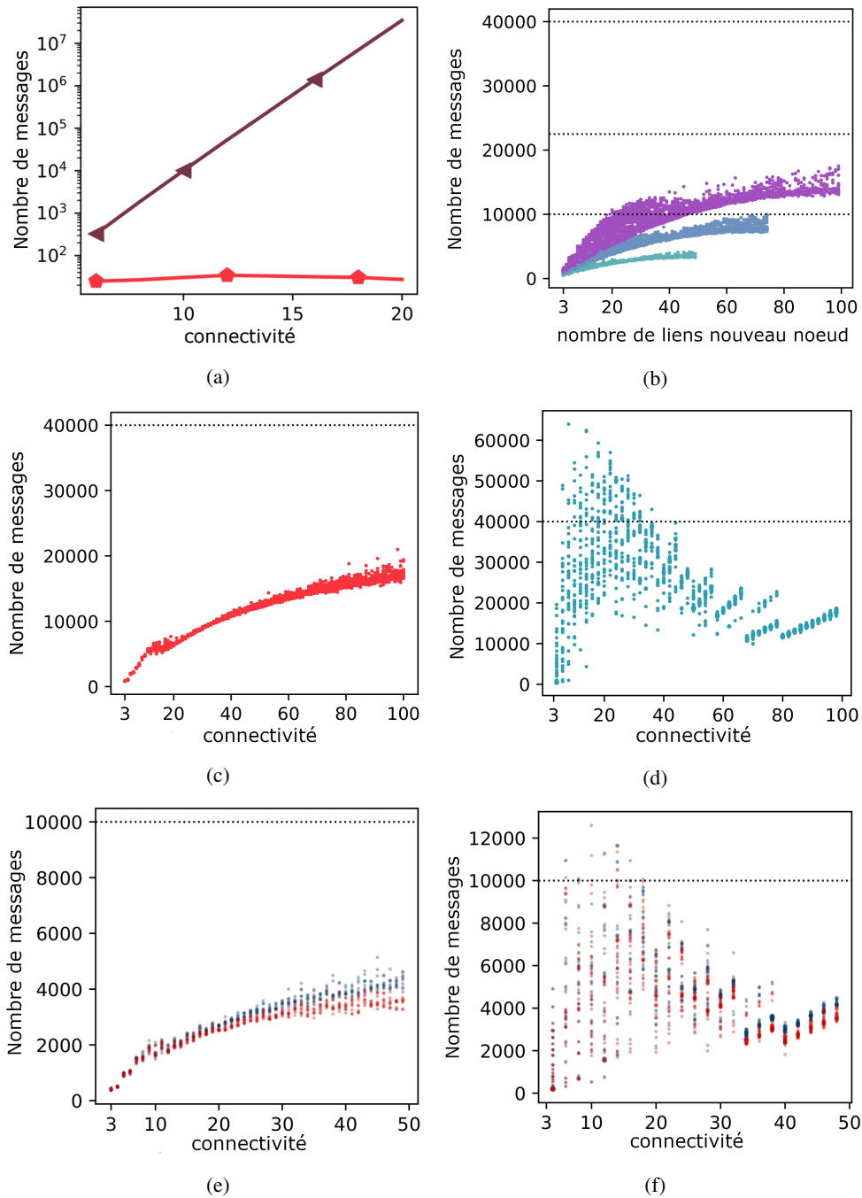
FIGURE 1: (a) graphe aléatoire k -régulier, comparaison entre Dolev (en marron) et le protocole modifié (en rouge), processus fautifs silencieux ; (b) graphe Barabási-Albert, n = 100, 150, 200 (respectivement de bas en haut), protocole modifié, processus fautifs silencieux ; (c) graphe aléatoire k -régulier k -connexe, n = 200 , protocole modifié, processus fautifs silencieux ; (d) roue multipartite, n = 200 , protocole modifié, processus fautifs silencieux ; (e) graphe aléatoire k -régulier k -connexe, n = 100 , protocole modifié, processus fautifs silencieux (en bleu) et actifs (en rouge) ; (f) roue multipartite, n = 100 , protocole modifié, processus fautifs silencieux (en bleu) et actifs (en rouge). Pour les figures (b)-(f), la ligne horizontale pointillée réfère à un nombre quadratique de messages échangés.
