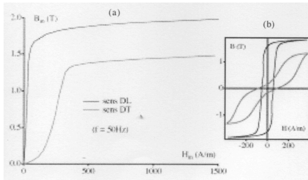
Figure 3: Fe-3%Si GO (a) courbes d'aimantation (b) cycles d'hystérésis caractéristiques, sens DL et DT.
