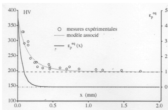
Figure 5: évolution corrélée de la dureté et de la déformation plastique en bord de découpe
