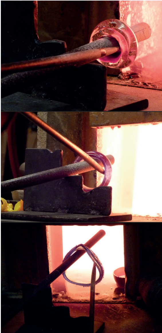
Fig. 2 Agrandissement d'une perle en bracelet avec deux ferrets. Avec un second outil inséré dans l'intérieur de la perle, le verrier exerce des pressions contrôlées sur tout le pourtour de l'anneau. L'agrandissement dépend du contrôle de la température et de la plasticité du verre, l'opération doit être réalisée devant le four. Trop chaud, l'anneau se déforme (en bas), trop froid, il ne s'agrandit pas (© J. Rolland).
