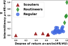
Figure 3: Privamov
