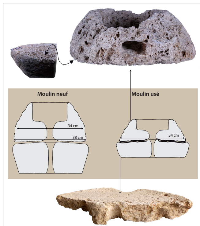
Fig. 15. Usures liées au profil tronconique et schémas interprétatifs. Clichés et schémas S. Lepareux-Couturier ; infographie N. Gomes.
