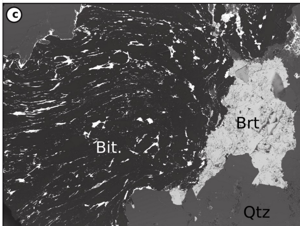
Mikouloungou (SEM-BSE)
