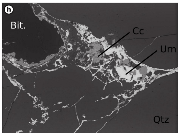
Mikouloungou (SEM-BSE)
