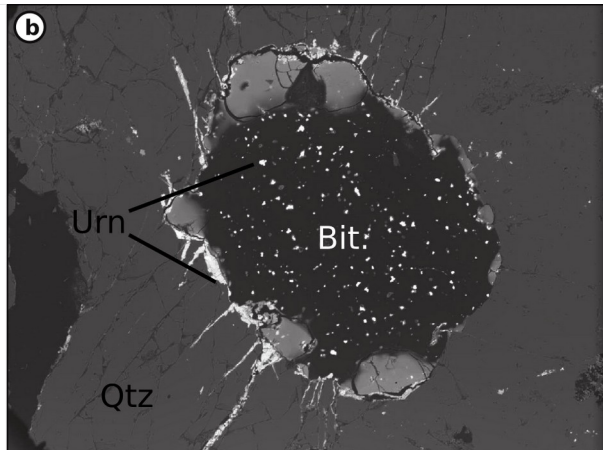
Bangombé (SEM-BSE)
