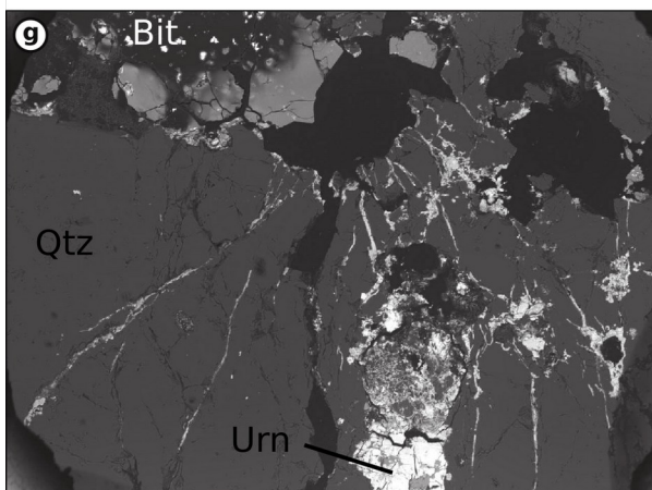
Bangombé (SEM-BSE)
