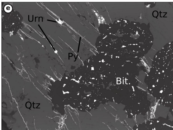
Okélobondo (SEM-BSE)
