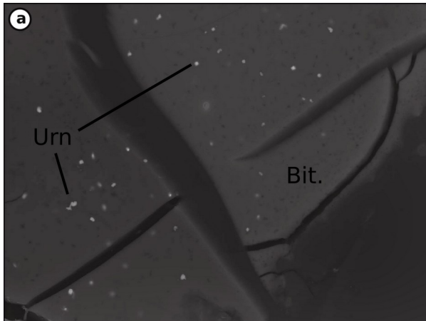
Nord Leyou (SEM-BSE)
