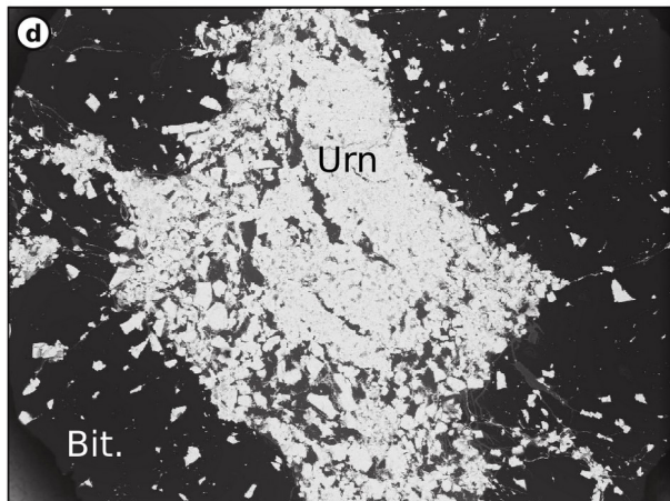
Okélobondo (SEM-BSE)
