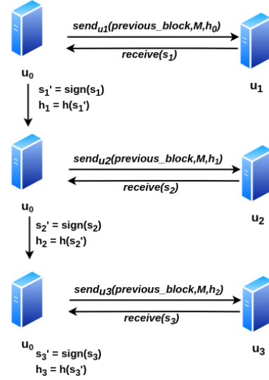
FIGURE 2: u_0 interagit de manière séquentielle avec les différents nœuds.
