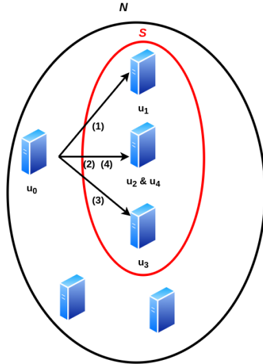
FIGURE 1: u_0 interagit avec un sous ensemble S de N
