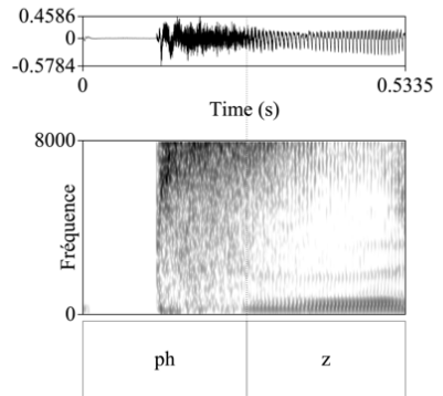
FIGURE 4 : Le signal acoustique et le spectrogramme de la forme /p h zʌ/, produite par FS1.
