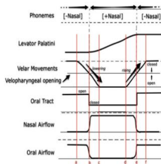
FIGURE 4 : Représentation schématique de la coordination aérodynamique et articuloire de la réalisation d'une nasale (Clements et al. (2014))
