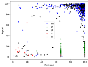
(d) occ_eval NEWSPAPER
