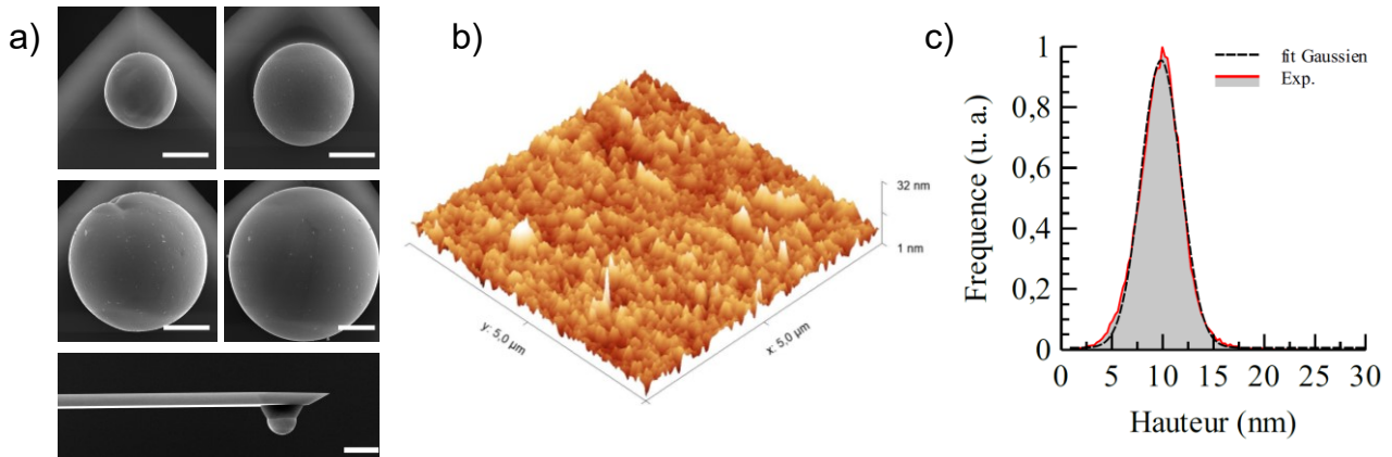
Figure 1 – Micrographies MEB des particules de tungstène greffées sur les leviers AFM (échelle 5 µm). Cartographie 3D de la surface en verre obtenue par AFM et histogramme des hauteurs des aspérités accompagné d'un ajustement gaussien
