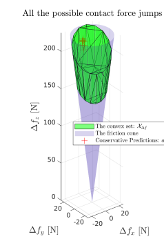
(d) Contact force
