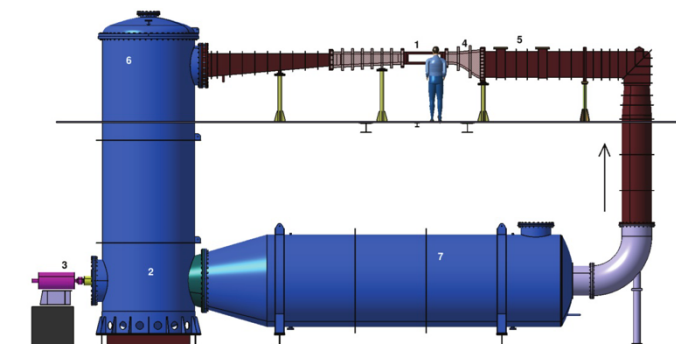
Figure 2. Vue schématique du tunnel hydrodynamique de l'IRENav, figure extraite de [3]
