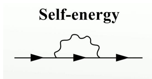
Fig. (1) Feynman Diagram
