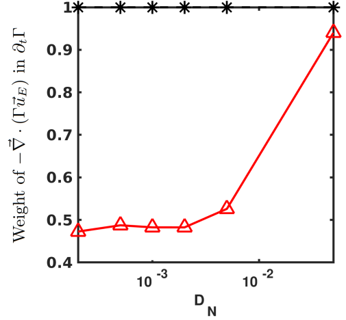
(d) Weight of -\vec{\nabla} \cdot (\Gamma \vec{u}_E) in \partial_t \Gamma .
