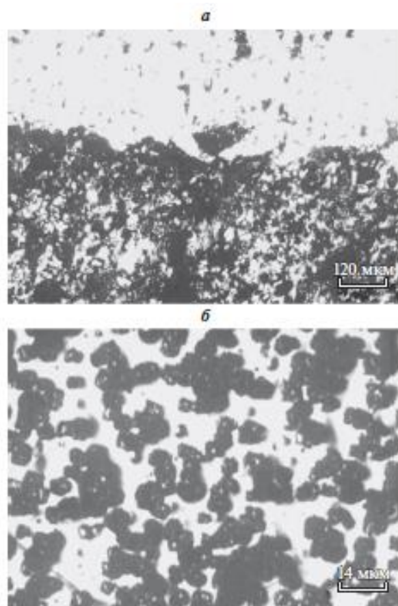
Рис. 20. Структура сплава Al–20 ат. % In, закристаллизованного со скоростью охлаждения V = 1 К/с от температур, лежащих (а) внутри области существования метастабильной микрогетерогенности (перегрев над ликвидусом \Delta T = 70 К) и (б) за пределами этой области ( \Delta T = 600 К).
