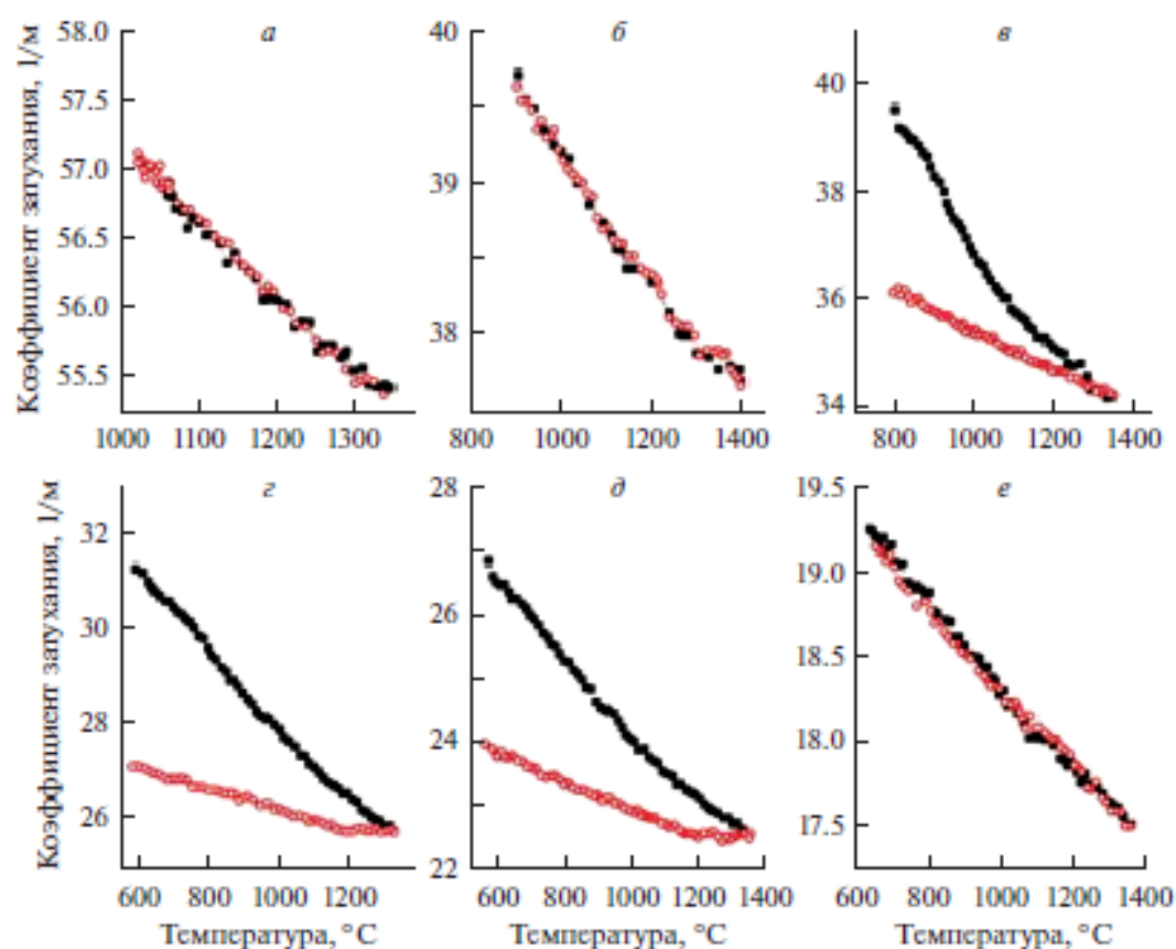
Рис. 18. Температурные зависимости произведения \rho\alpha некоторых сплавов Al–Cu: (а) \text{Al}_5\text{Cu}_{95} , (б) \text{Al}_{45}\text{Cu}_{55} , (с) \text{Al}_{55}\text{Cu}_{45} , (д) \text{Al}_{75}\text{Cu}_{25} , (е) \text{Al}_{95}\text{Cu}_5 при нагреве (сплошные символы) и последующем охлаждении (пустые символы).
