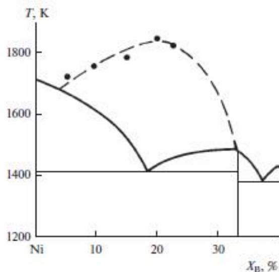
Рис. 3. Фазовая диаграмма системы Ni–В. Пунктирная линия над ликвидусом ограничивает область метастабильной микрогетерогенности расплавов.
