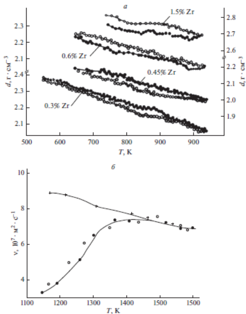
Рис. 13. (а) Температурные зависимости плотности расплавов Al-Zr ( \circ – нагрев, \bullet – охлаждение; концентрация циркония дана в ат. %) и (б) температурные зависимости вязкости лигатуры Al-2 мас. % Zr ( \bullet – первый нагрев, + – охлаждение, \circ – повторный нагрев после затвердевания).
