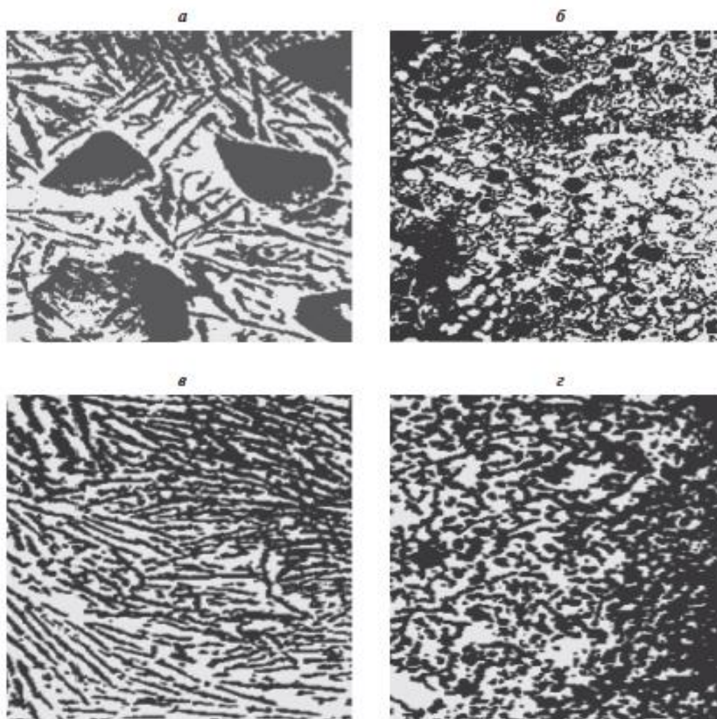
Рис. 12. Структура сплава Al–17 ат. % Si, выплавленного без гомогенизирующего перегрева и закристаллизованного со скоростями (а) 10^2 и (б) 10^{5^{\circ}}\text{C}/\text{с} , и после гомогенизирующей термической обработки в жидком состоянии и кристаллизации со скоростями (в) 10^2 и (г) 10^{5^{\circ}}\text{C}/\text{с} ( \times 200 ) [26].
