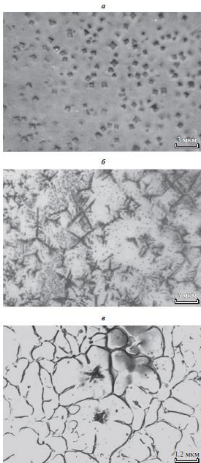
Рис. 16. Трансформация форм роста кристаллов алюминидов циркония (структура типа L1_2 ) в зависимости от перегрева исходного расплава ( V = 10^4 К/с): (а) \Delta T = 100 К; (б) \Delta T = 300 К; (в) \Delta T = 450 К.
