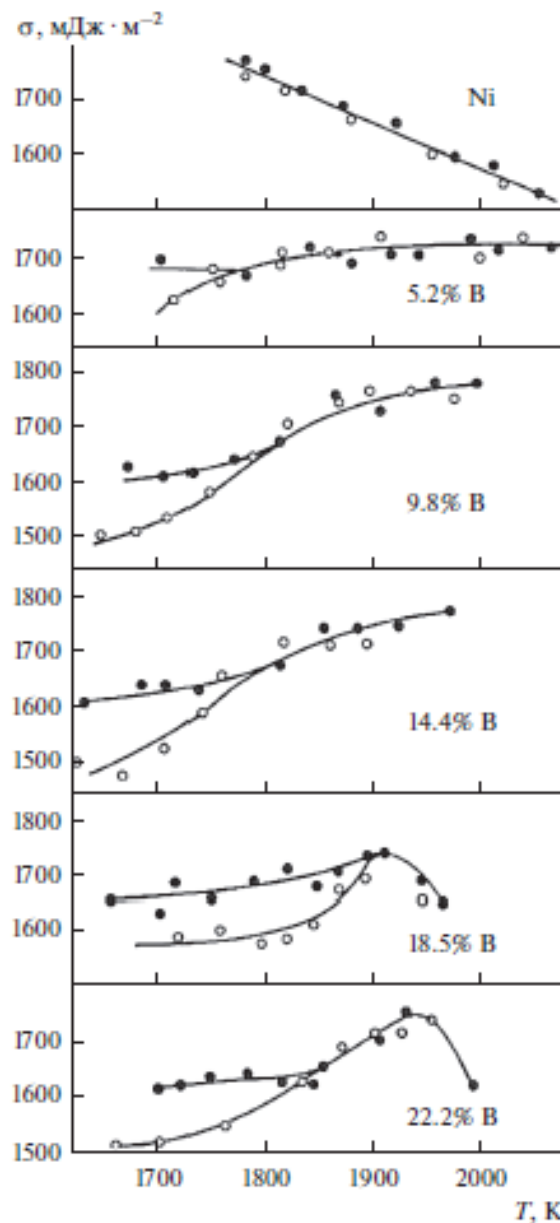
Рис. 2. Температурные зависимости поверхностного натяжения расплавов Ni–B, полученные при нагреве после плавления (●) и при последующем охлаждении (○).
