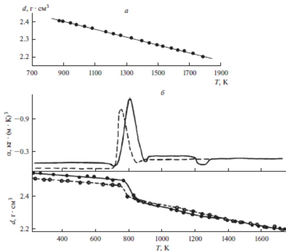
Рис. 10. (а) Температурные зависимости плотности, полученные при охлаждении расплава Al–Si эвтектического состава, приготовленного при 1450°C и (б) температурные зависимости плотности и коэффициента термического расширения, полученные после плавления этого образца (●, ○ обозначают экспериментальные данные, полученные при нагреве и охлаждении этого образца соответственно; линии представляют собой сглаживающий сплайн и его производную).
