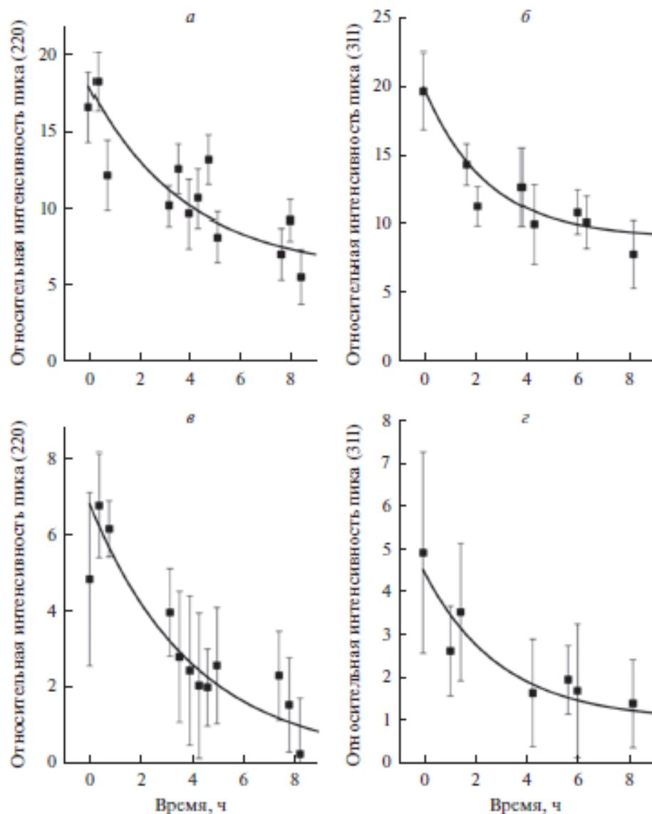
Рис. 9. Изменения со временем дифракционных пиков Ni (220) и (311): пик (220) при температуре 904 (а) и 952°С (в); пик (311) при 904 (б) и 952°С (з). Кривые получены как результат экспоненциальной аппроксимации экспериментальных данных.
