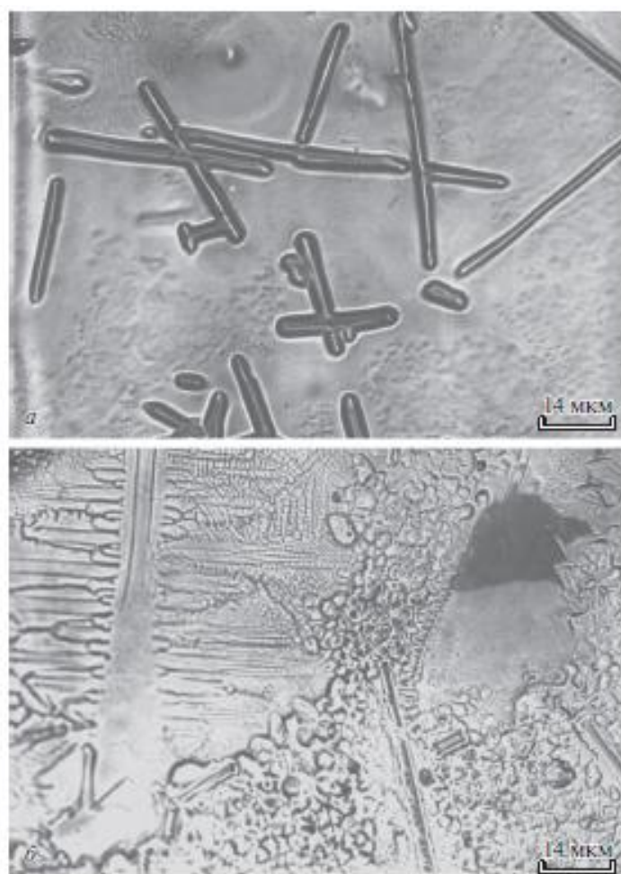
Рис. 14. Формы роста кристаллов алюмината циркония (структура типа D0_{23} ) в зависимости от параметров затвердевания для сплава Al–2 мас. % Zr: (а) V = 10 К/с, \Delta T = 200 К; (б) V = 10^3 К/с, \Delta T = 360 К.
