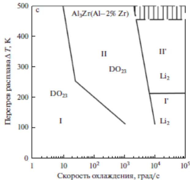
Рис. 15. Области роста кристаллов с различной морфологией алюминидов циркония (I – огранные кристаллы; II – дендритные кристаллы).
