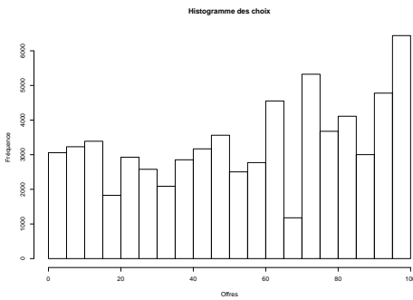
FIGURE 2 – Choix réalisés via l'algorithme partial pooling de THOMPSON-SAMPLING.
