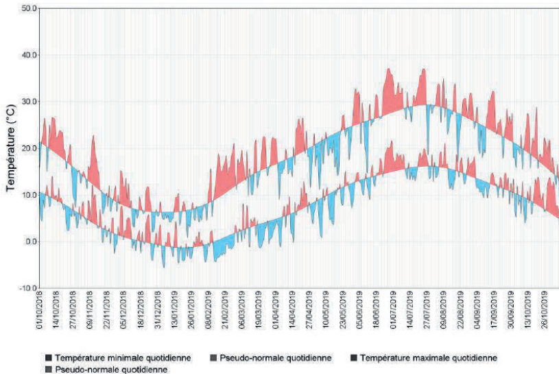
Figure 2 : Températures quotidiennes maximales et minimales à Grenoble sur plus d'un an, du 1 er octobre 2018 au 7 novembre 2019, comparées à la moyenne de 30 années antérieures (1980-2010). Source : Météo-France
