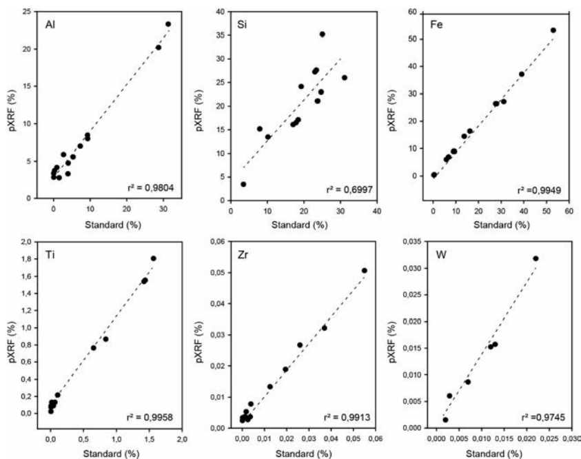
FIGURE 5 – Droites d'étalonnages pour plusieurs éléments établies grâce au logiciel PyMca à partir des paramètres fondamentaux. Acquisitions réalisées par un instrument ELIO (XGlab), dans l'air, à une tension de 40 kV et un courant de 100 \mu A pendant 5 min.
