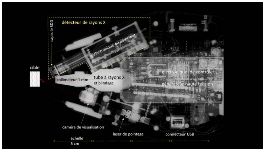
FIGURE 1 – Radiographie d'un appareil p-XRF (ELIO XGLab/Bruker). On distingue le détecteur de type SDD et le tube à rayons X en ligne miniature avec son collimateur de 1 mm, le pointeur laser et la caméra. La tête de mesure pèse 1.9 kg. © T. Calligaro, C2RMF
