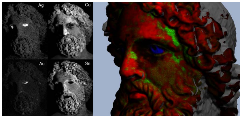
FIGURE 3 – A gauche, carte de répartition des composants du bronze et des incrustations : Cu, Sn, Ag, Au. La taille du faisceau est de 200\mu\text{m} . A droite, la cartographie 2D XRF a été reportée sur le scan 3D optique (Cu=rouge, Sn=vert, Ag=bleu). © C2RMF
