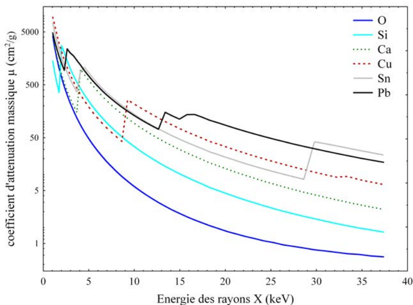
FIGURE 4 – Variation du coefficient d'atténuation massique \mu en fonction de l'énergie de rayons X et pour six éléments de numéro atomique croissant. On note que le coefficient \mu varie sur plusieurs ordres de grandeur.
