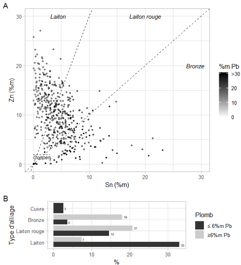
FIGURE 10 – A - Graphique représentant les taux de zinc (Zn) en fonction des taux d'étain (Sn) exprimés en % massique. Les zones correspondantes à chaque type d'alliage sont délimitées par des lignes en pointillés en fonction de la nomenclature proposée par [54] : Cuivre non allié < 3\%m\ Sn et < 2\%m\ Zn , Laiton Zn \geq 3Sn\ \%m , Bronze Zn < Sn , Laiton rouge Sn \leq Zn \leq 3Sn\ \%m . B - Histogramme de distribution des objets selon les types d'alliages qui les composent.
