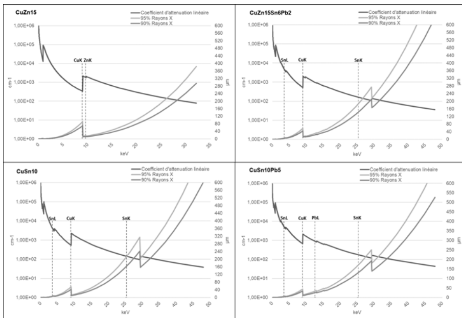
FIGURE 9 – Coefficients d'atténuation linéaire de quatre alliages à base de cuivre (CuZn15, CuZn15Sn6Pb2, CuSn10, CuSn10Pb5) et profondeurs spécifiques d'origine du signal détecté en fonction de l'énergie. Les barres verticales indiquent les énergies des transitions K ou L des éléments de l'alliage.
