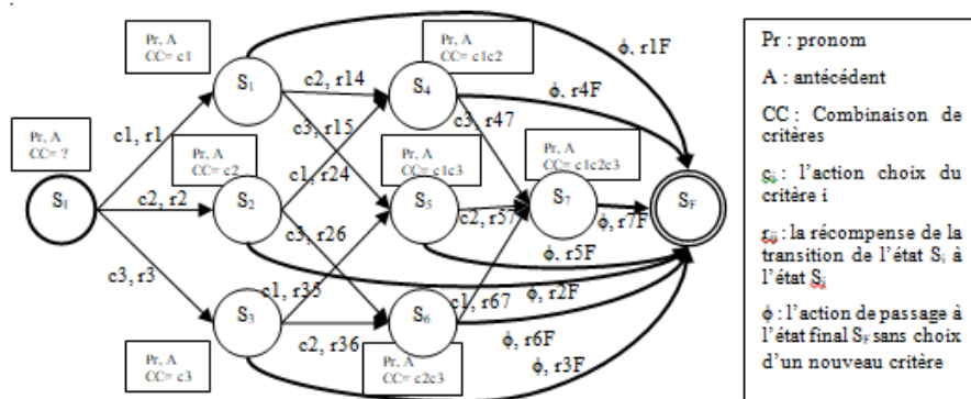
FIGURE 2 : Modélisation PDM pour la résolution des pronoms
