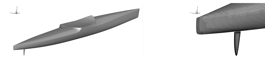
FIGURE 10 – (a) Vue générale de la configuration avec dérive; (b) zoom autour de la dérive avec le maillage de surface.
